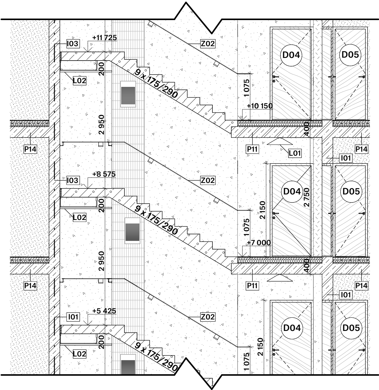
Řezopohled C-C'
