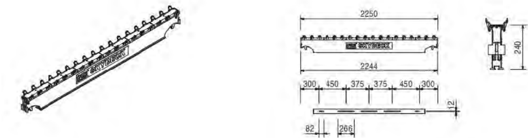
Obrázek: nosník STL 225
