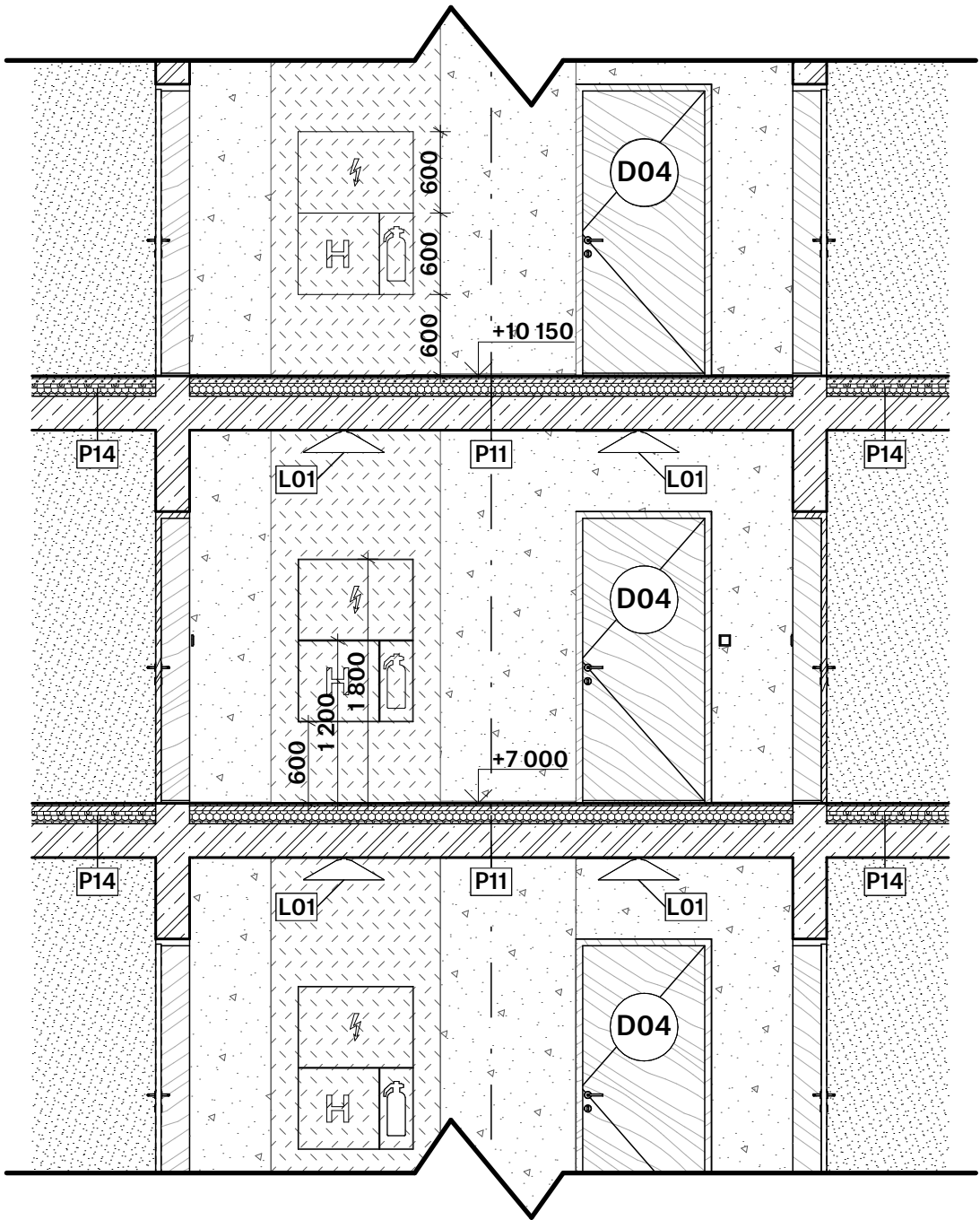
Řezopohled D-D'
