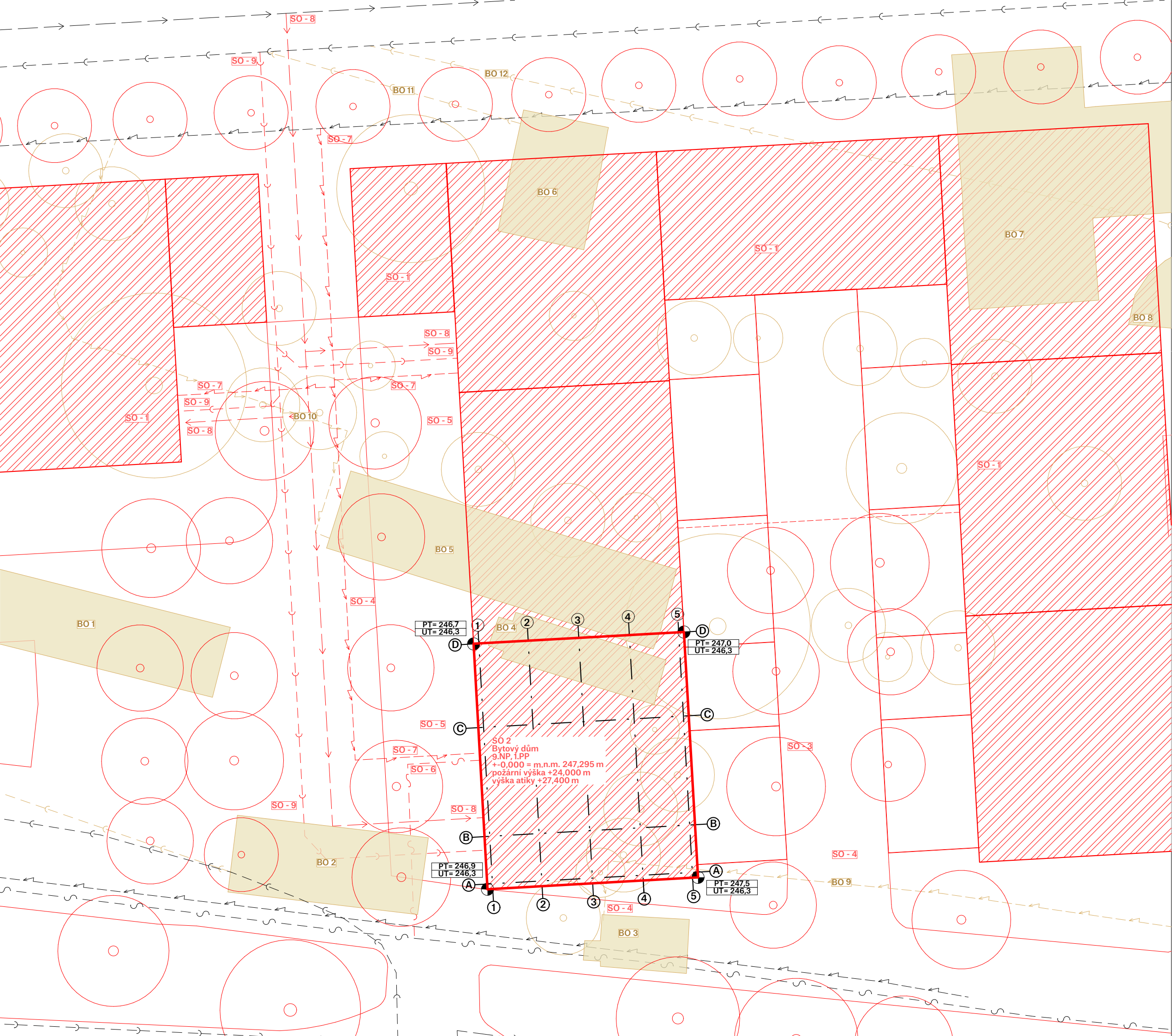
M 1:3000 schéma bytového souboru
