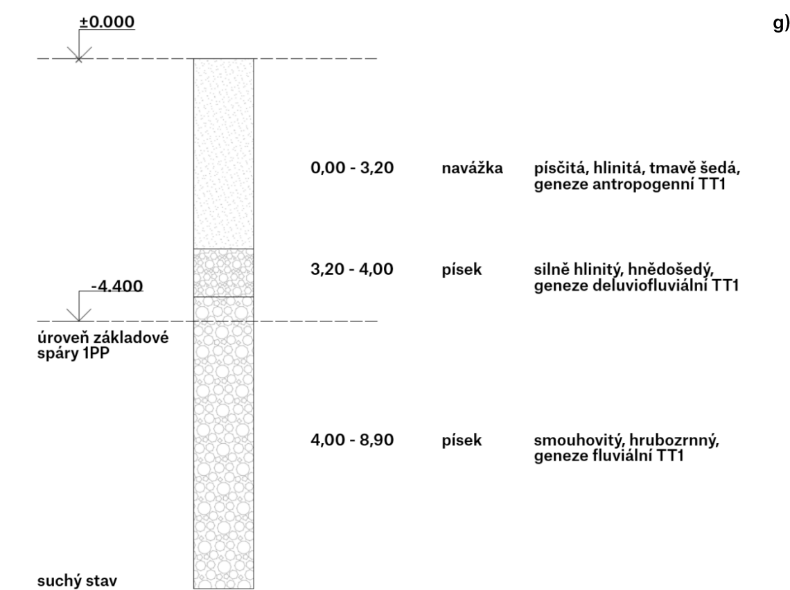
Obrázek 2 – Geologický vrt
