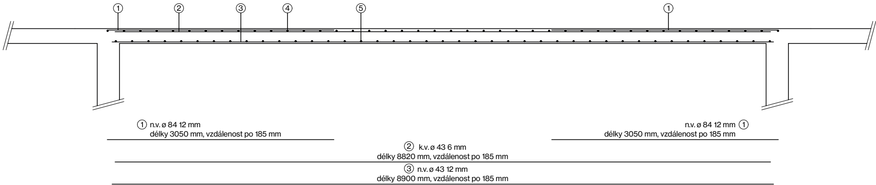
ŘEZ A-A'
