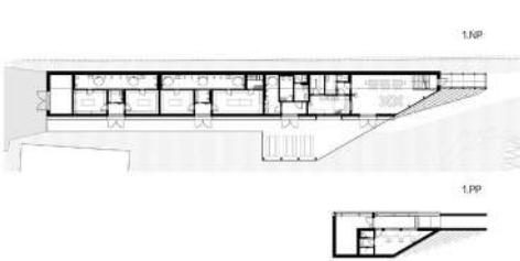
půdorys fotbalového zázemí, autoři Chrama, Studenec, Česká republika, 2021
