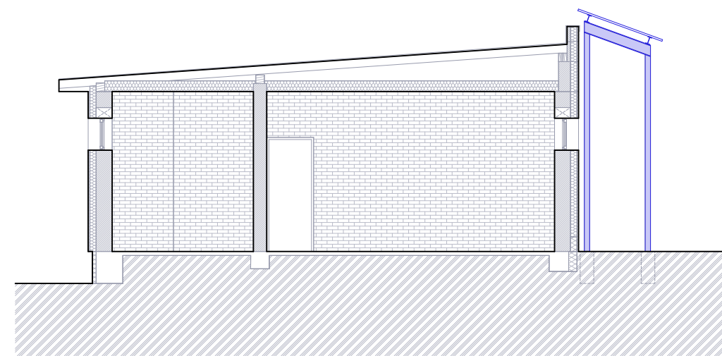
řez D-D
