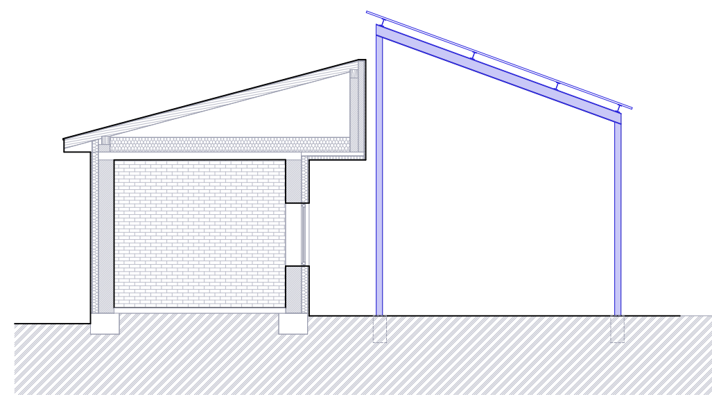
řez B-B
