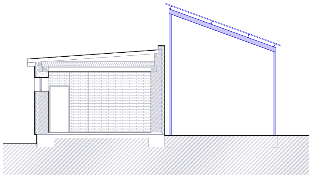
řez A-A
