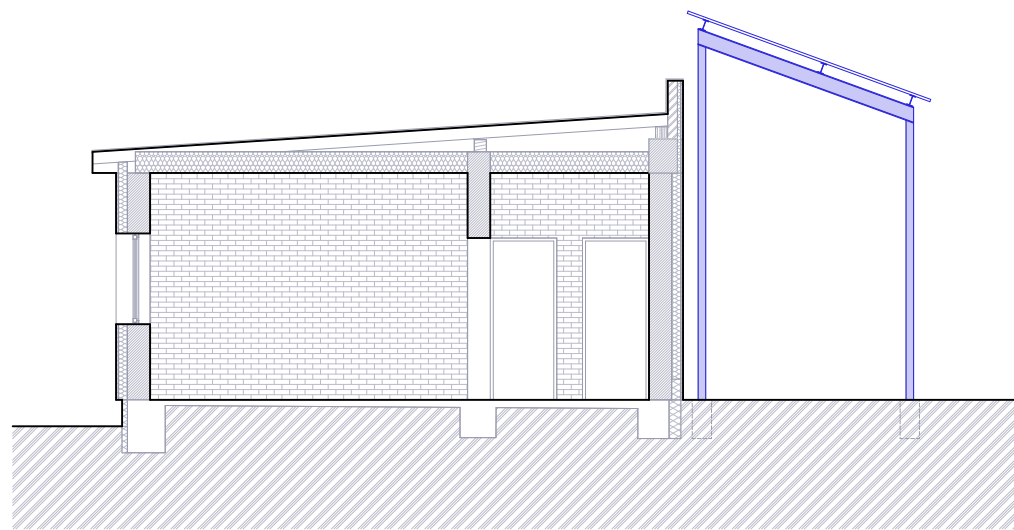
řez C-C
