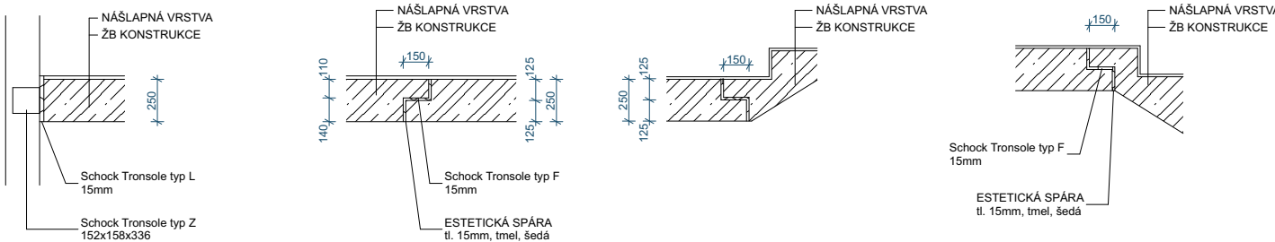
Uložení prefabrikátu M 1:20
