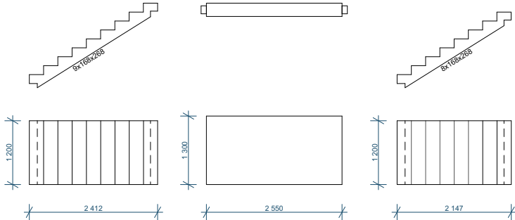
Výpis prefabrikátu M 1:50
