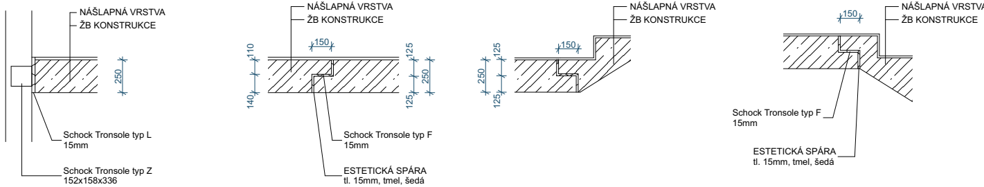
Uložení prefabrikátu M 1:20
