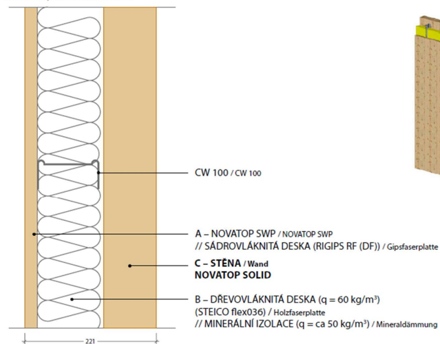
Vodorovný řez / Horizontalschnitt
