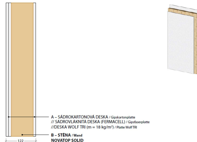
Vodorovný řez / Horizontalschnitt
