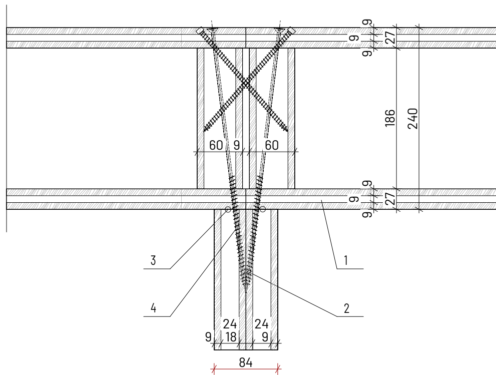
DETAIL ULOŽENÍ DVOU STROPNÍCH PANELŮ NA NOSNOU STĚNU
