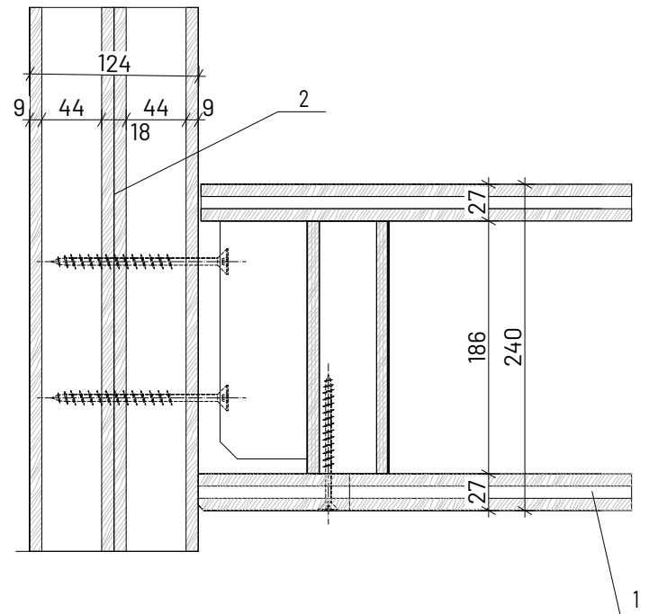
DETAIL ULOŽENÍ STŘEŠNÍHO PANELU POMOCÍ OCELOVÉHO L PROFILU
