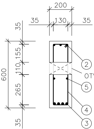
ŘEZ C–C'
