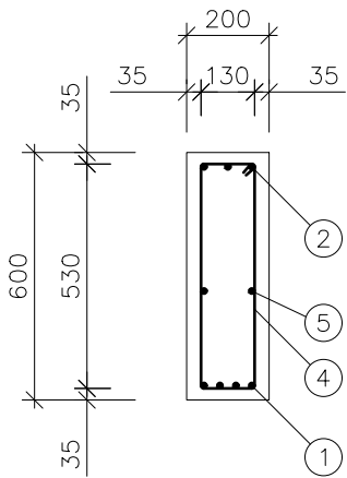
ŘEZ A–A'
