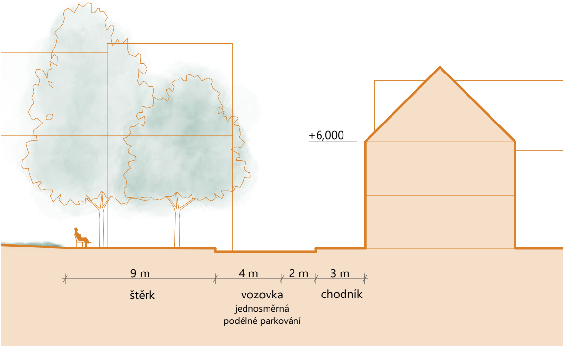
ULIČNÍ PROFIL - JIŽNÍ STRANA NÁMĚSTÍ
