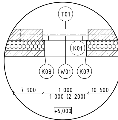
PR. 2. PŮDORYSNÝ ŘEZ V ÚROVNI 2,3m NAD PODLAHOU
