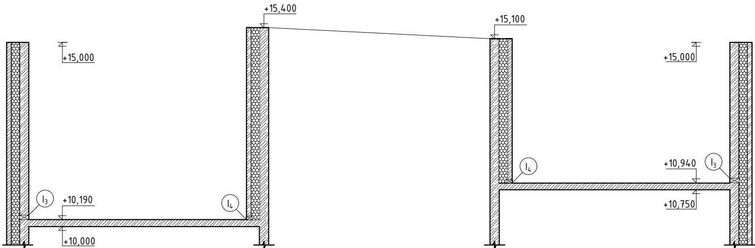
ŘEZ - B''
