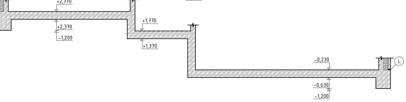
ŘEZ - C
