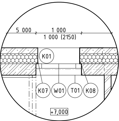
PR. 1. PŮDORYSNÝ ŘEZ V ÚROVNI 2,2m NA PODLAHOU
