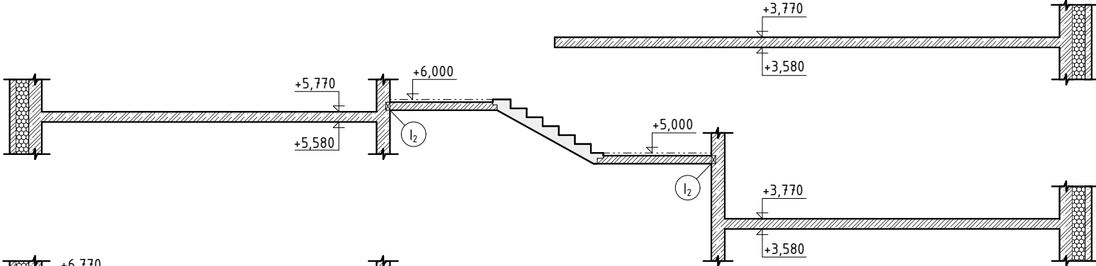
ŘEZ - B'
