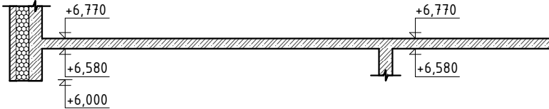
ŘEZ - A'
