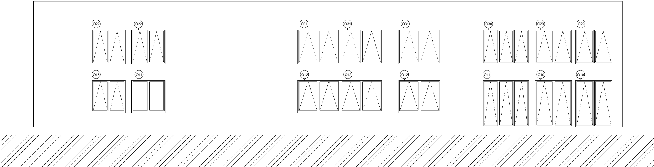
Západní pohled
