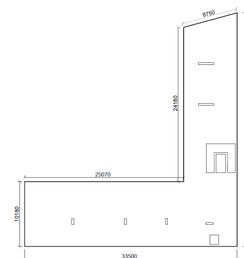
Zdroj: vlastní výkres vodorovné nosné kce
