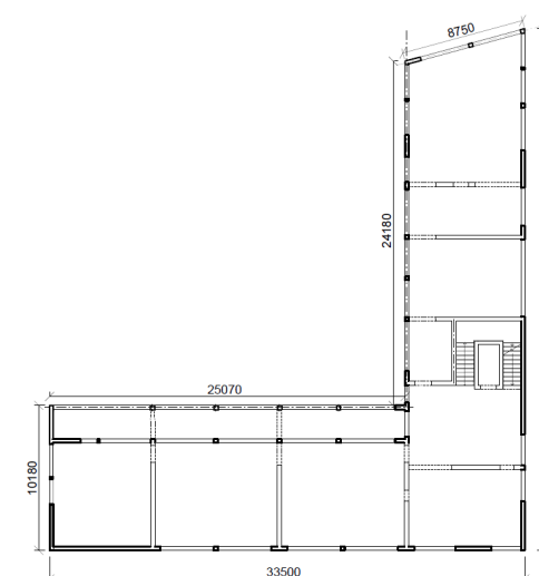
Zdroj: vlastní výkres svislé nosné kce
