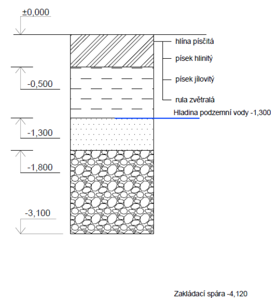
Obrázek č.2, Náčrt složení půdy, Zdroj [2]
