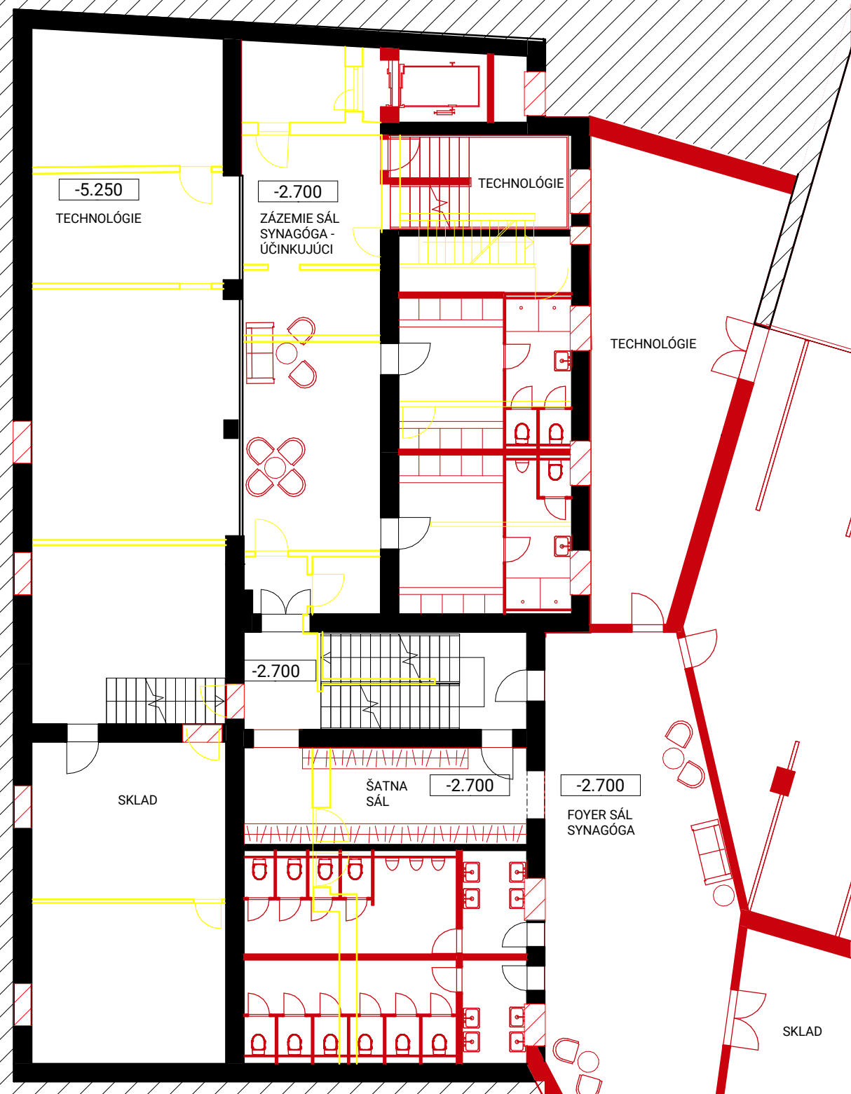
1PP KULTÚRNE CENTRUM 1:150
