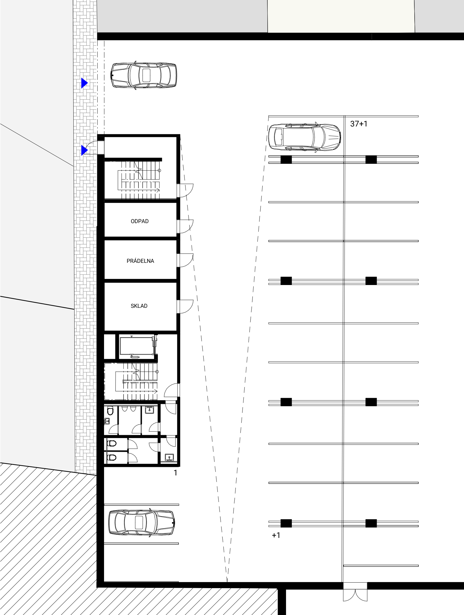
1PP HOTEL 1:150
