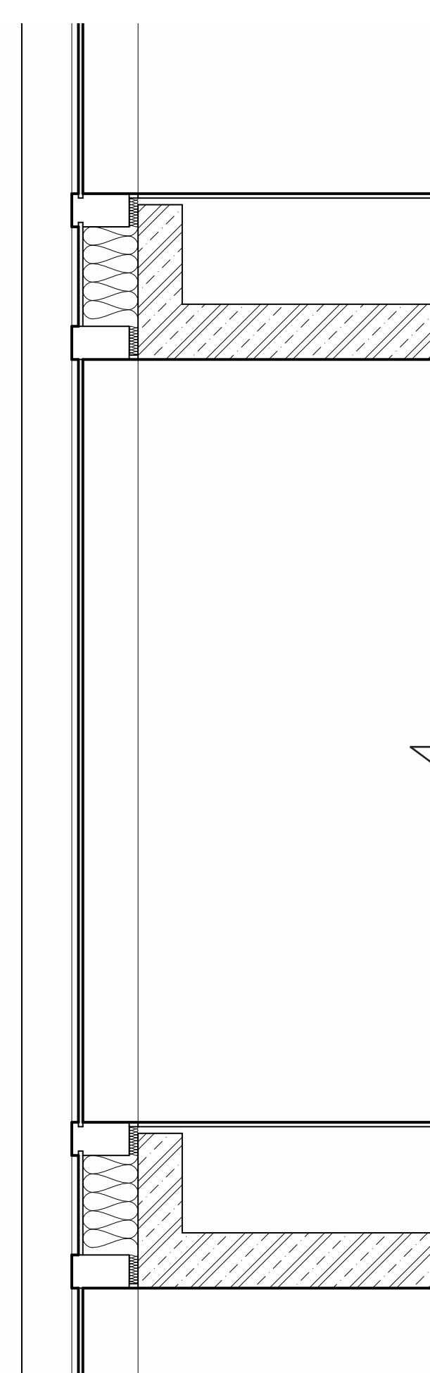
DETAIL KCE M1:25
