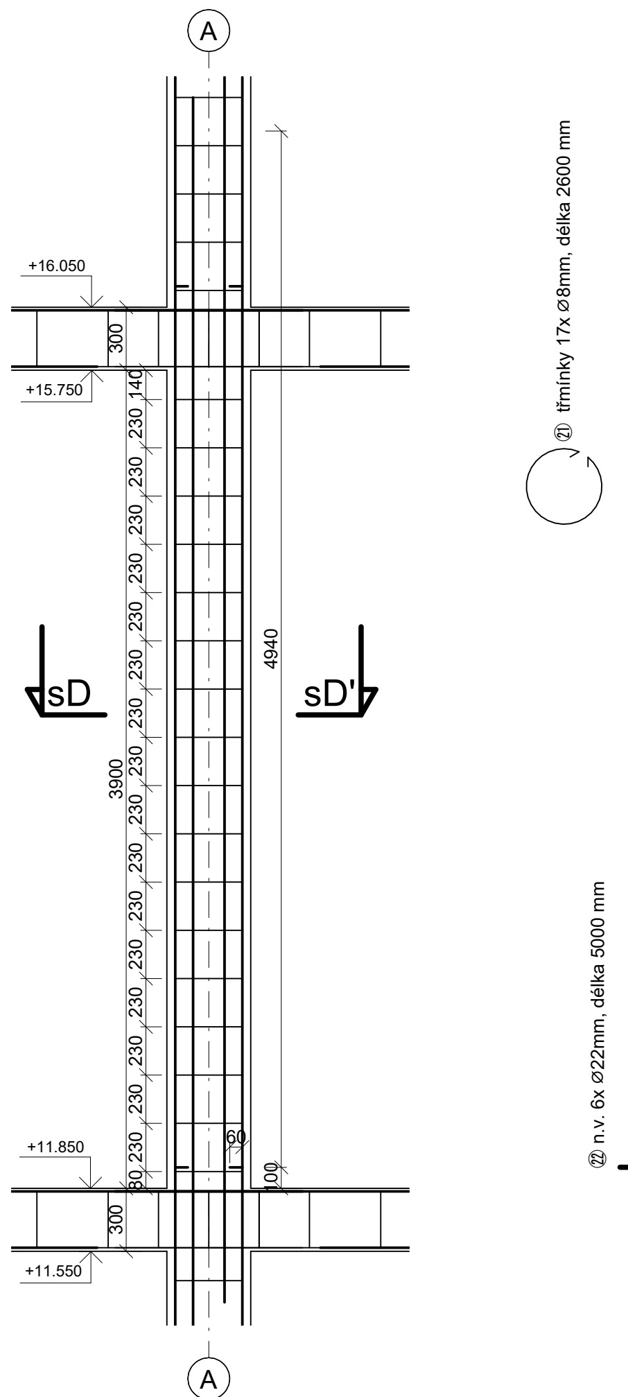
VÝKRES VÝZTUŽE SLOUPU 1:25
