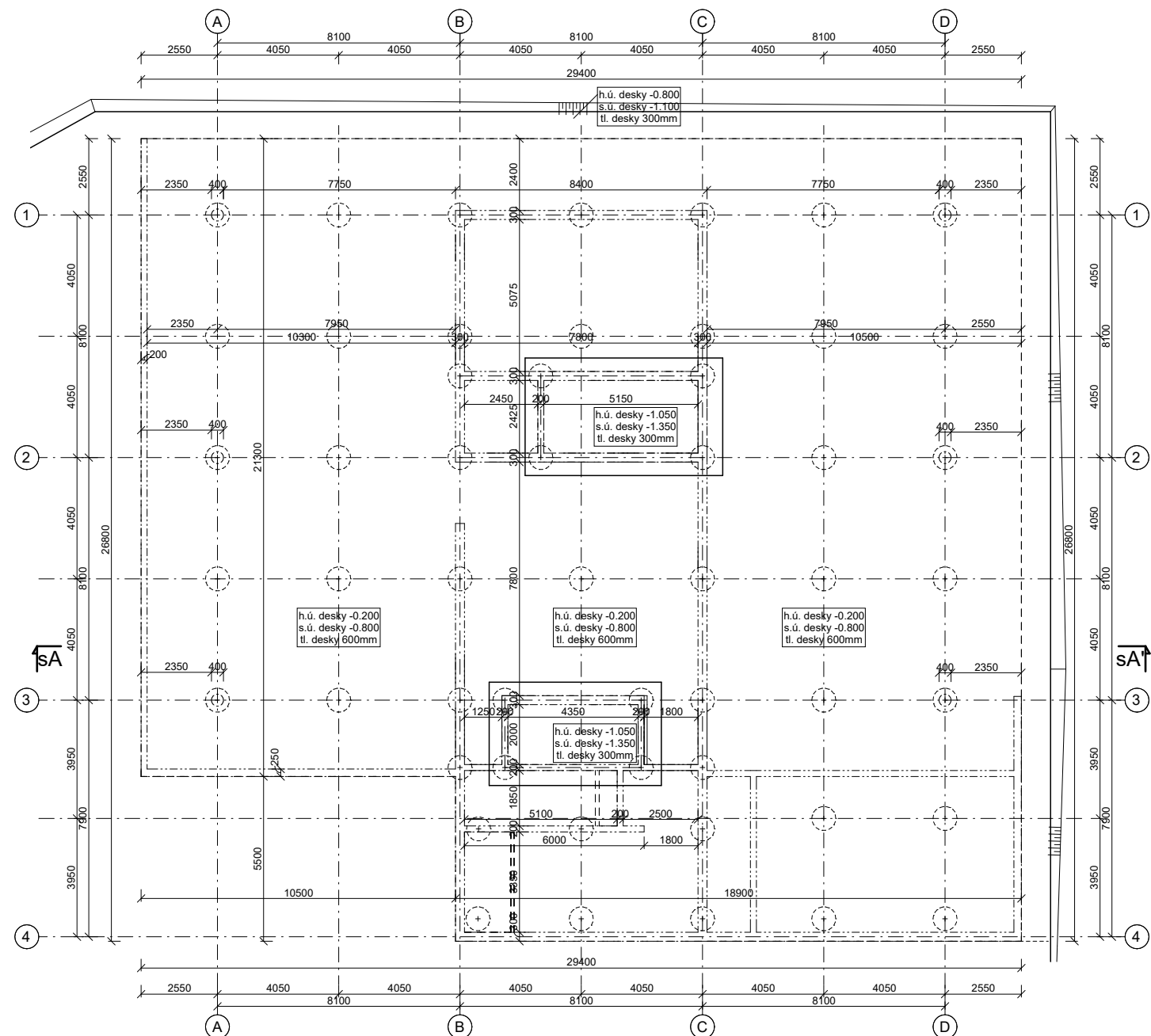
D.2.b.1 PŮDORYS ZÁKLADŮ 1 : 100
