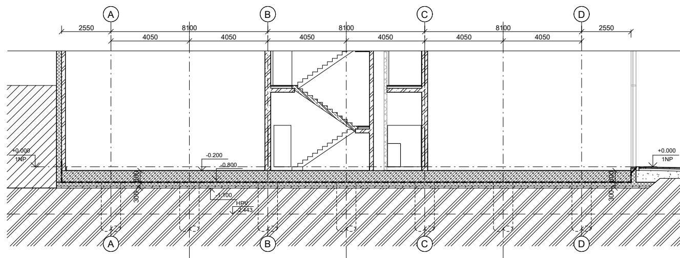
D2b1 ŘEZ ZÁKLADY 1 : 100
