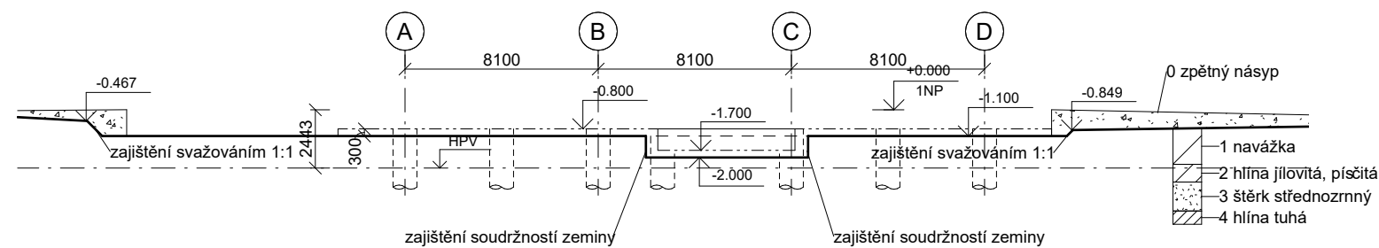
D.5.b.2 ŘEZ rA-A' STAVEBNÍ JÁMA 1 : 200
