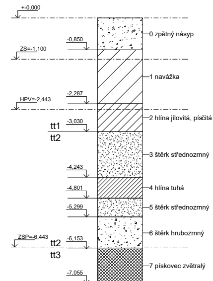
PŮDNÍ PROFIL (INT. 19056 & 568160)
