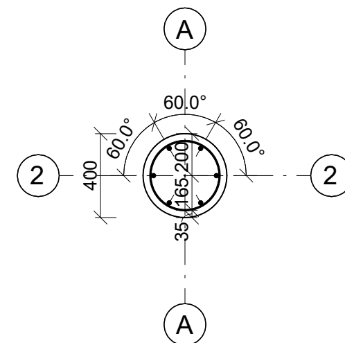
PŮDORYSNÝ ŘEZ G-G' 1:25
