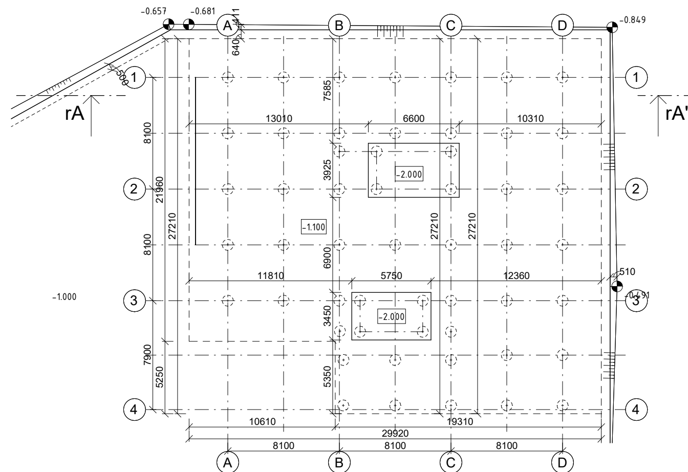
D.5.b.2 STAVEBNÍ JÁMA 1 : 200
