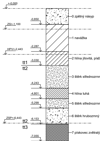
PŮDNÍ PROFIL 1:50 (INTERPOLACÍ 19056 & 568160)
