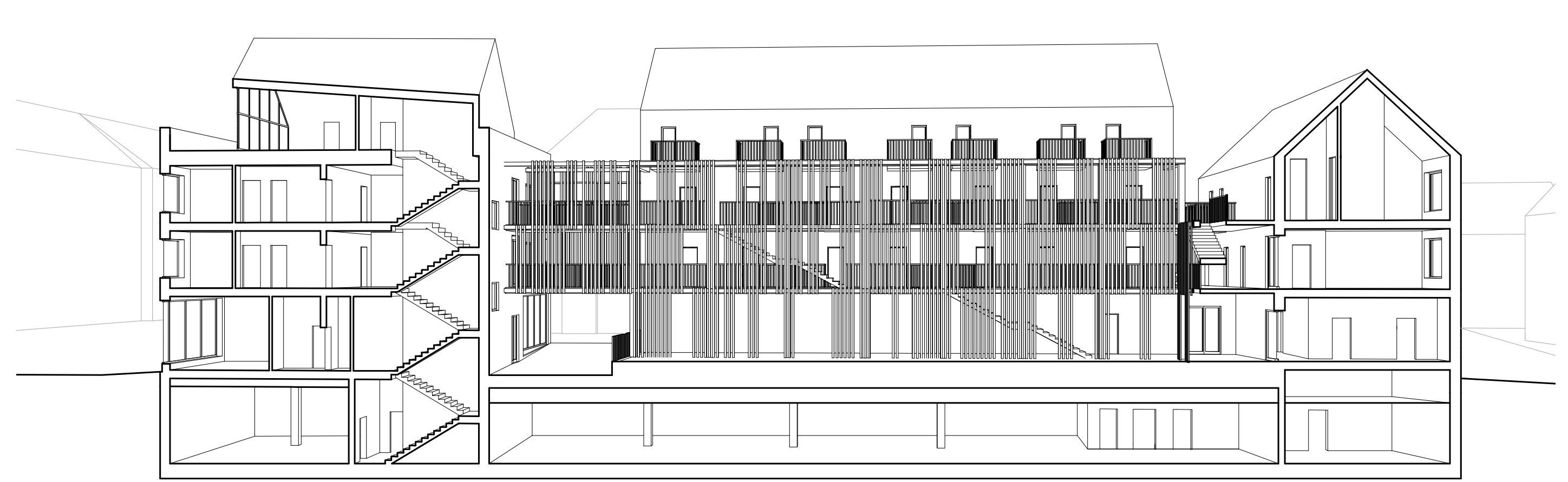
Řezopohled c-c, 1:200
