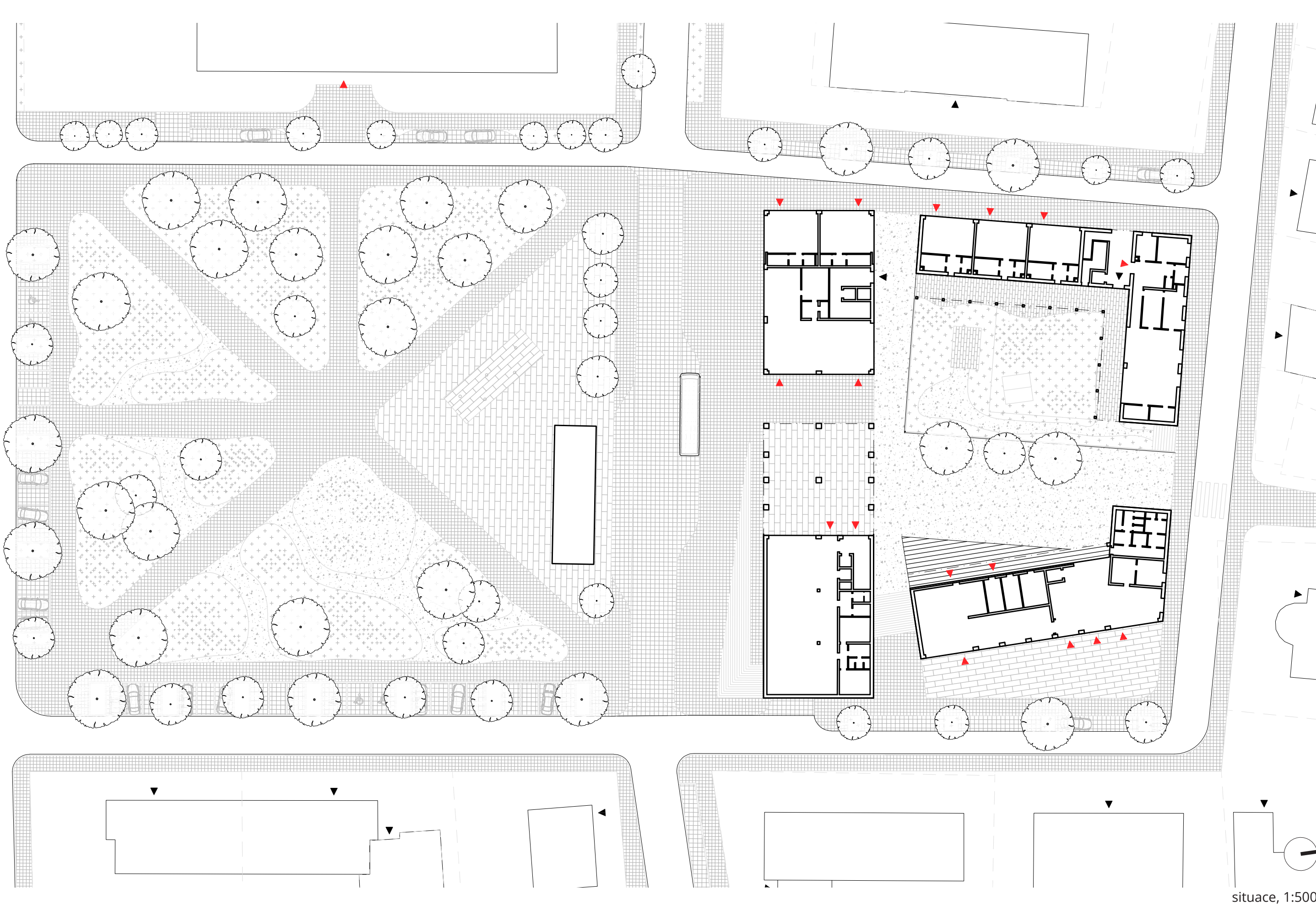
situace, 1:500
