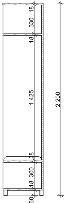
ŘEZ B - B' M 1:25
