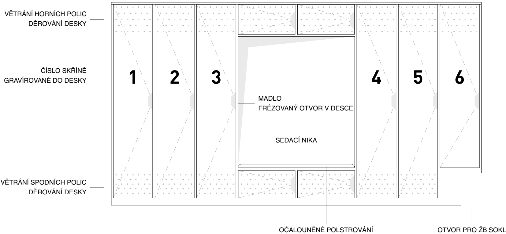
ČELNÍ POHLED M 1:25
