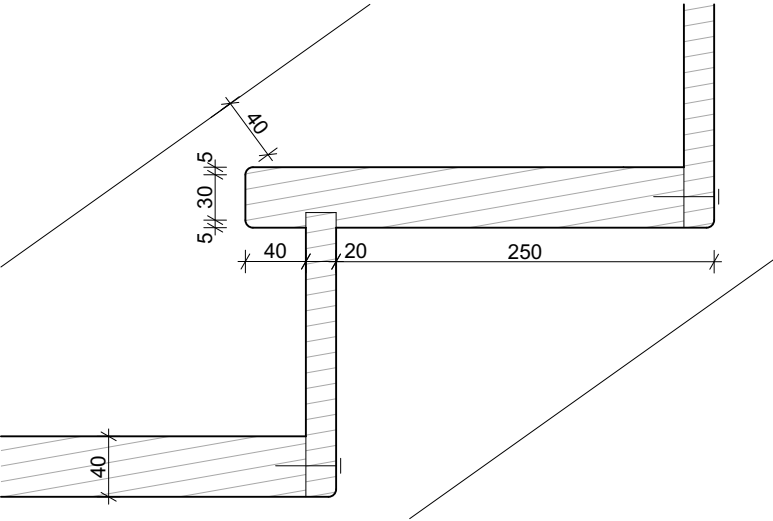
DETAIL SCHODIŠŤOVÝCH STUPŇŮ M1:5
