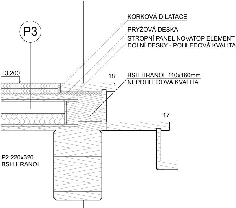
DETAIL ULOŽENÍ SCHODIŠTĚ VE 2.NP M1:10
