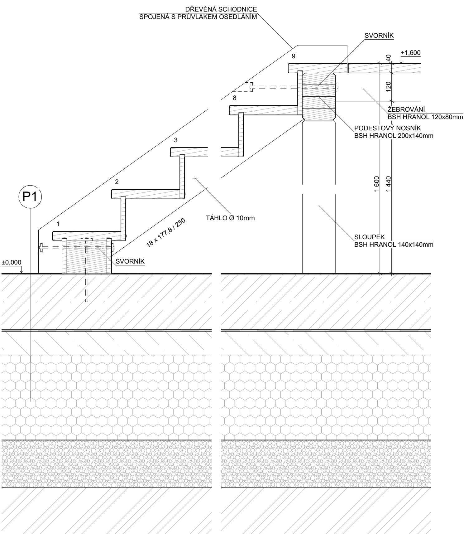
PODÉLNÝ ŘEZ SCHODIŠŤOVÝM RAMENEM M1:10
