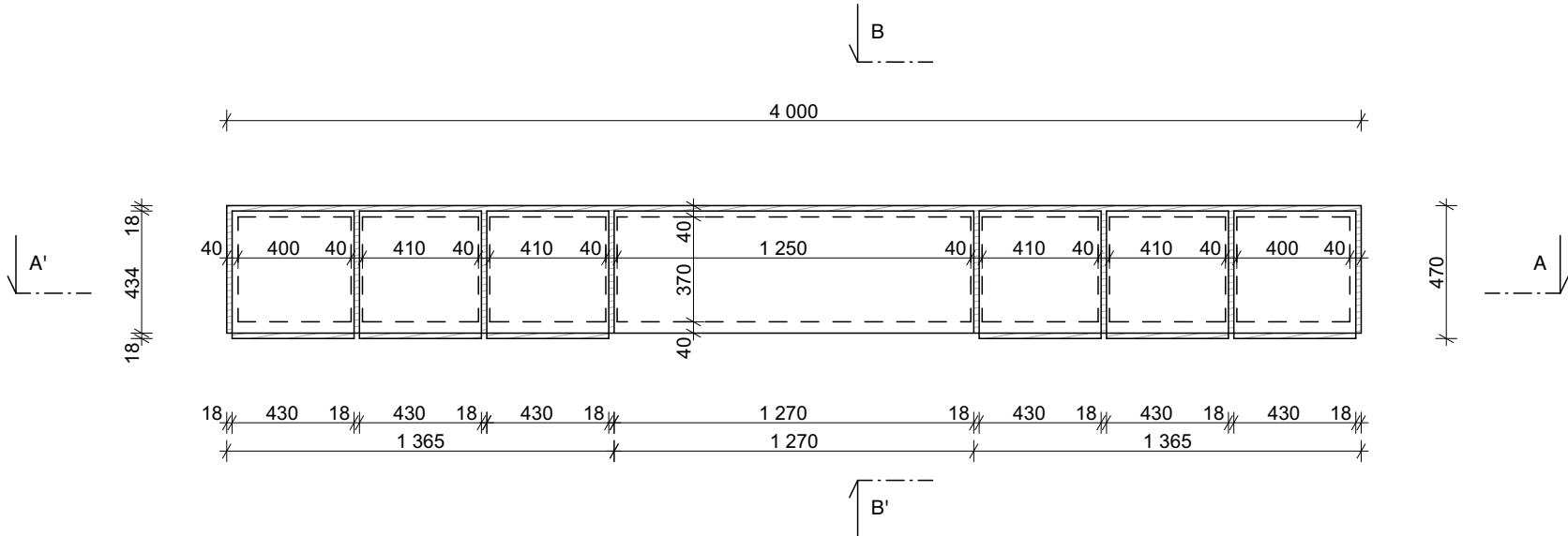
PŮDORYS M1:25
