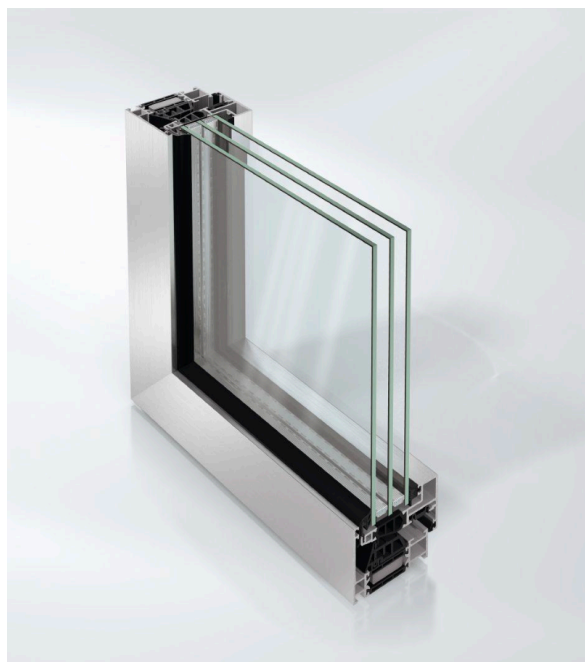
Schüco AWS 75 BS.HI+
