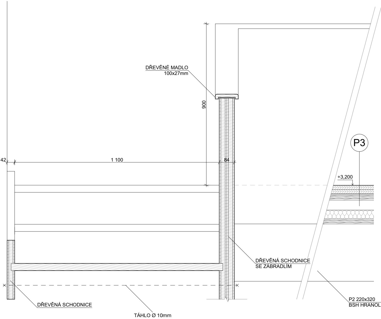
PŘÍČNÝ ŘEZ SCHODIŠŤOVÝM RAMENEM M1:10
