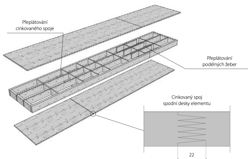
Obr. č. 2 - Standardní formáty panelů NOVATOP ELEMENT [6]
