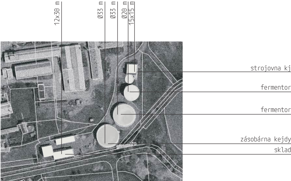
Bioplynová stanice Kněžice
