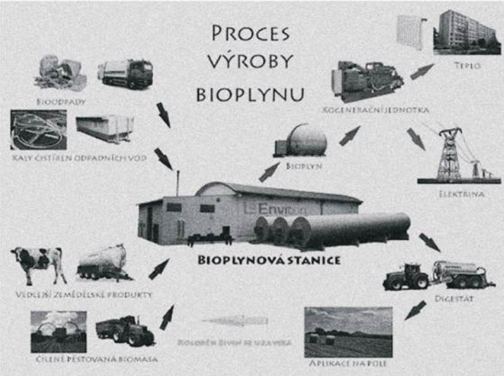
schéma procesů
