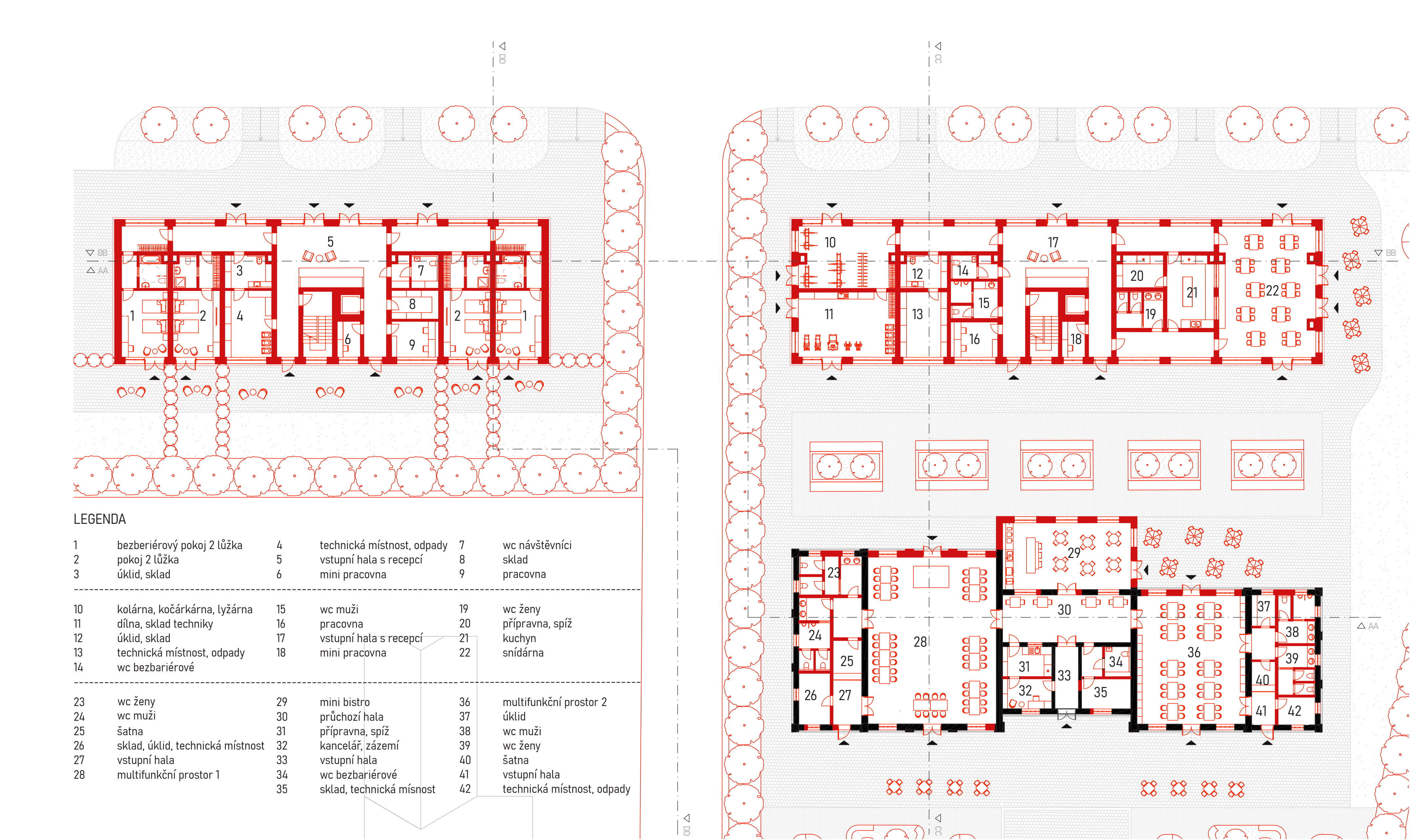
PŮDORYS _ 1NP
