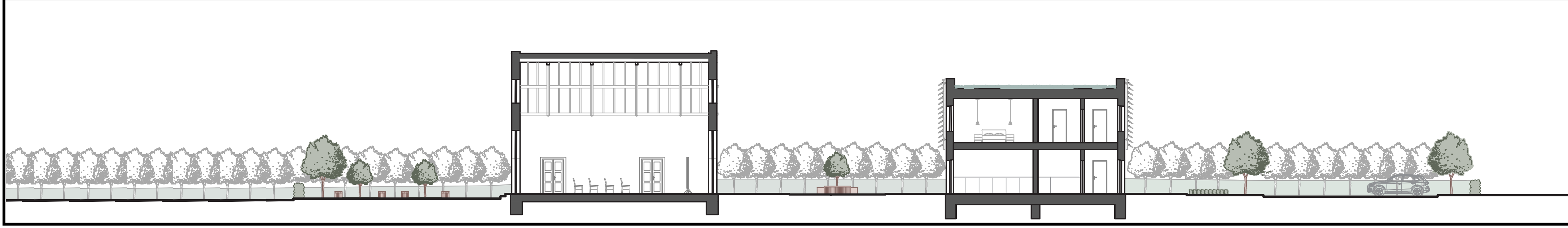
ŘEZ CC
