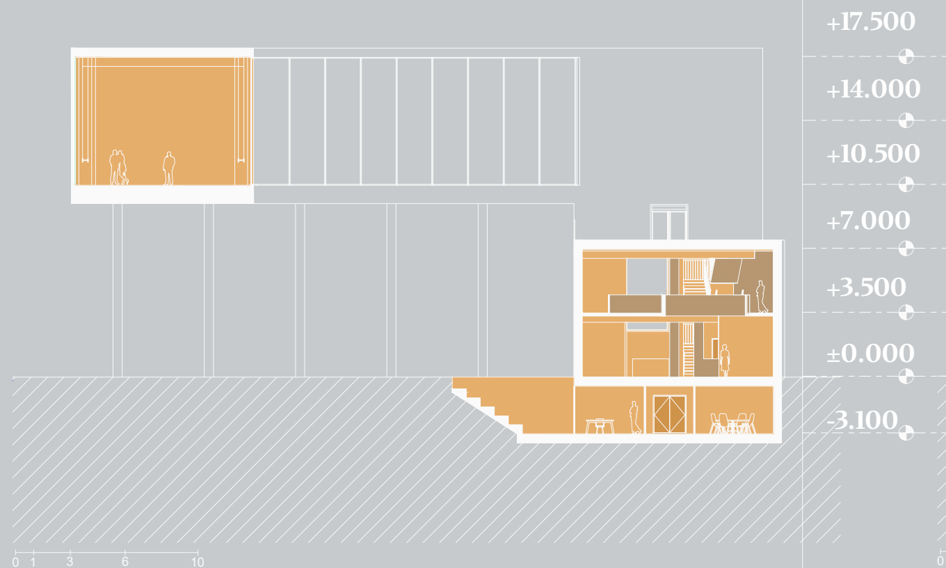
Řez 1-1
