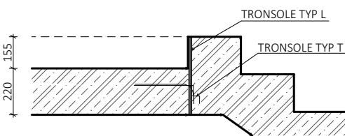
T3- NAPOJENÍ RAMENE NA STROPNÍ DESKU
