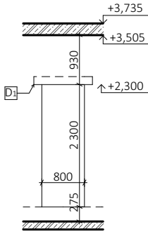
D1- OTVOR PRO DVEŘE
