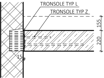
T1- NAPOJENÍ MEZIPODESTY A STĚNY
