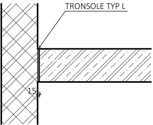
T2- DILATACE MEZI SCHODIŠTĚM A STĚNOU
