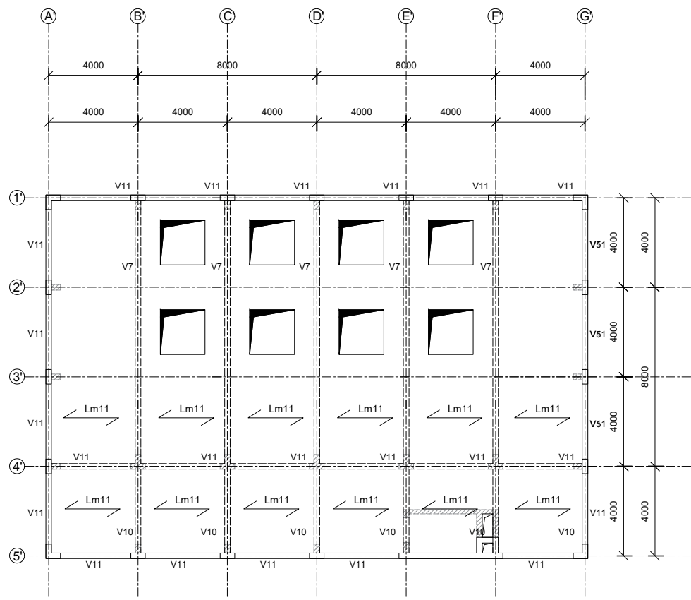
COBERTURA
