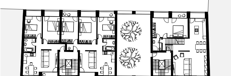
Půdorys 5zp
