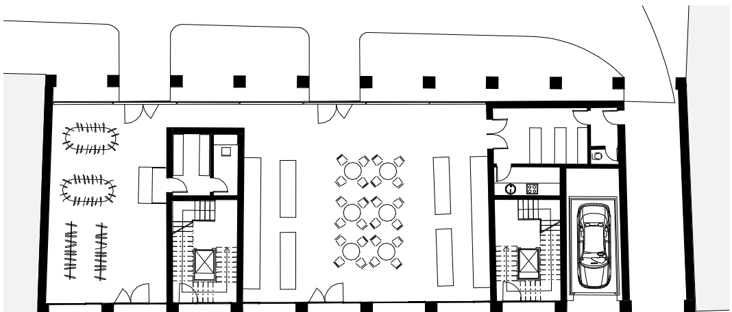
Půdorys parteru
