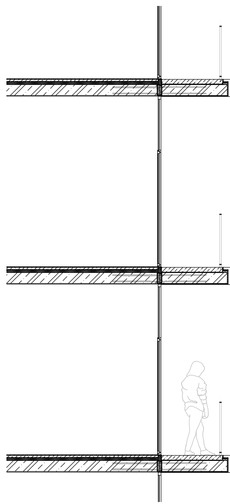
Řez A-A
