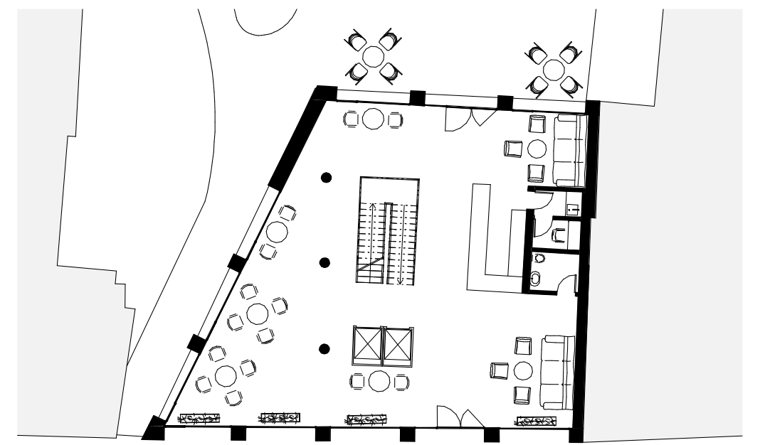
Půdorys parteru
