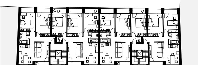
Půdorys 4zp-4np
