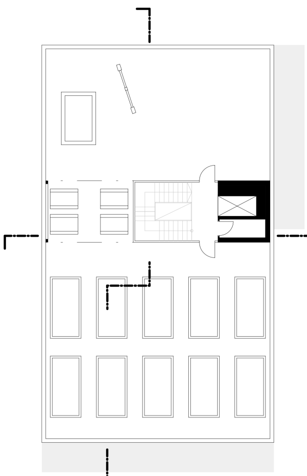
Pódozys střecha
