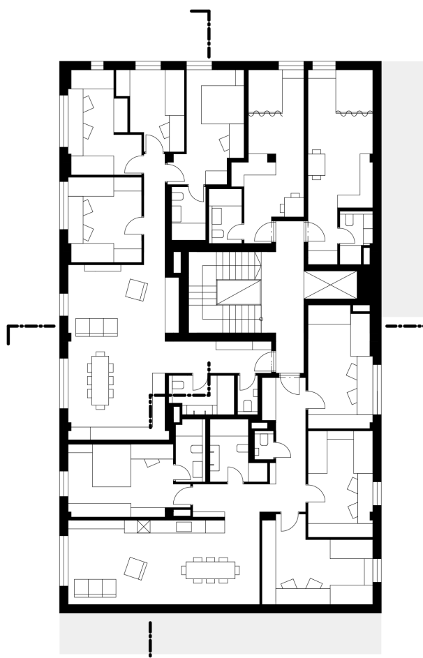
Pódozys 3.NP-6.NP
