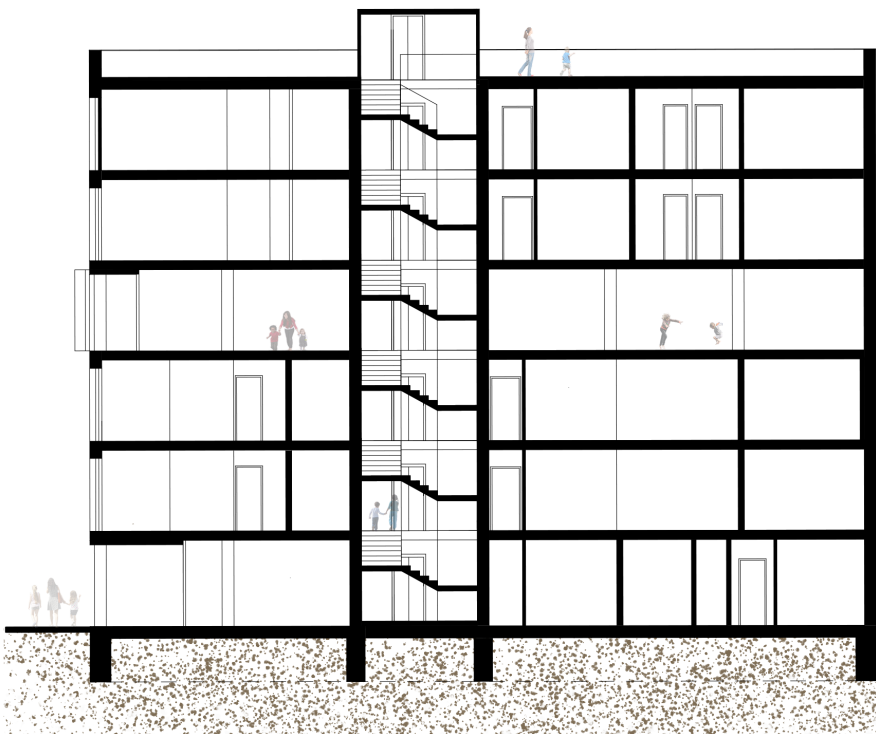
Rez podélný
