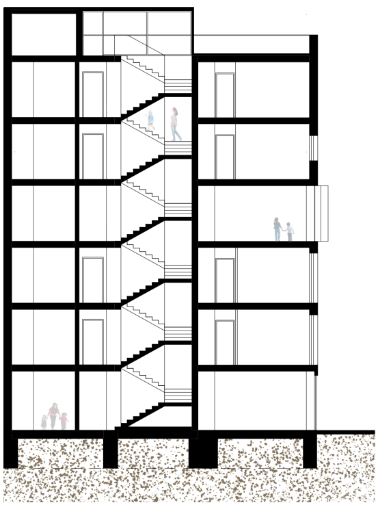
Rez příčný
