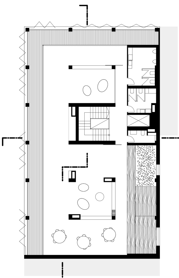
Pódozys 4.NP
