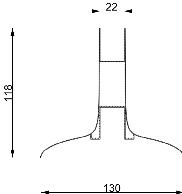
ŘEZ M 1 : 2
