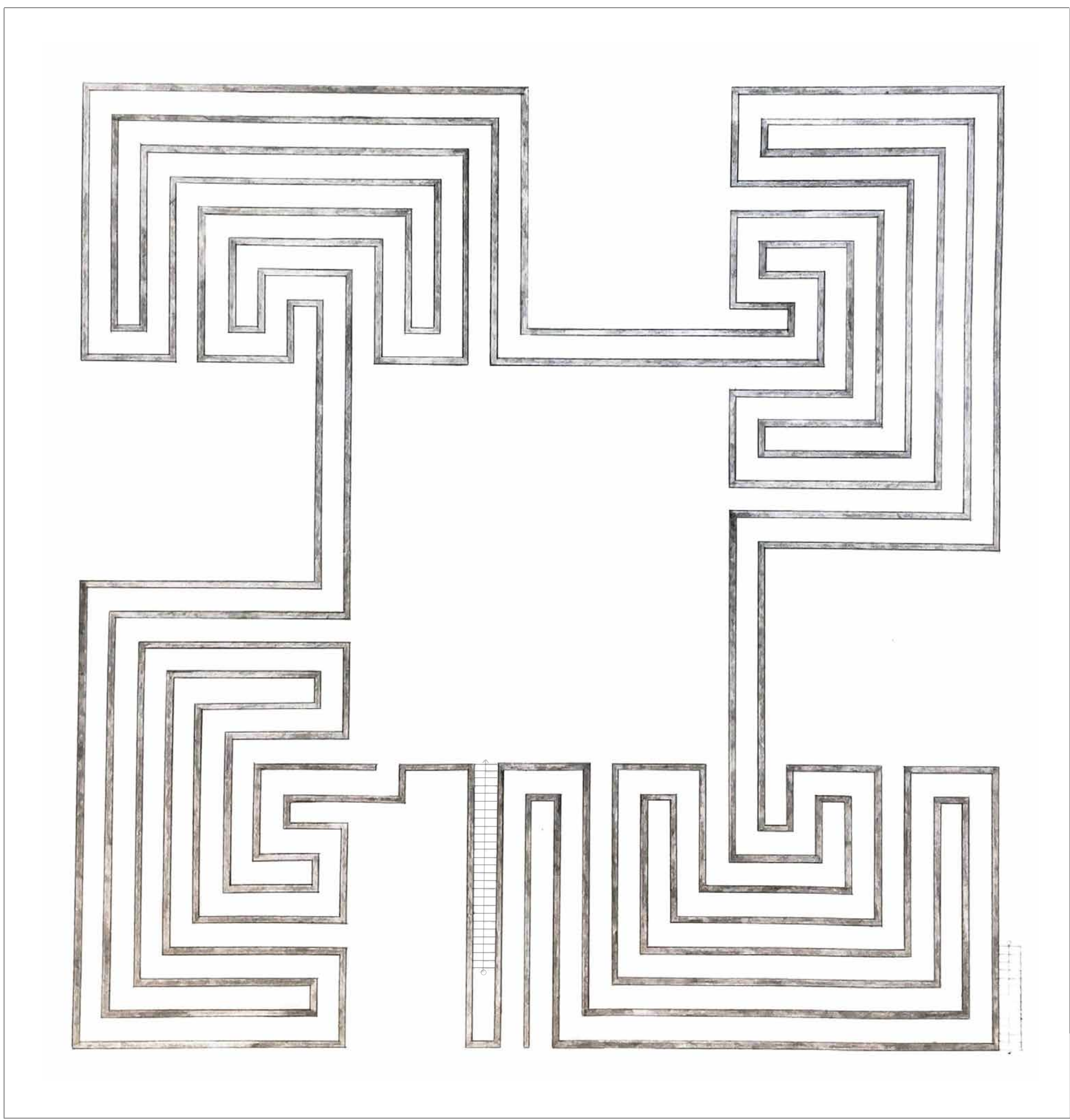
Púdorys 2NP 1:100
