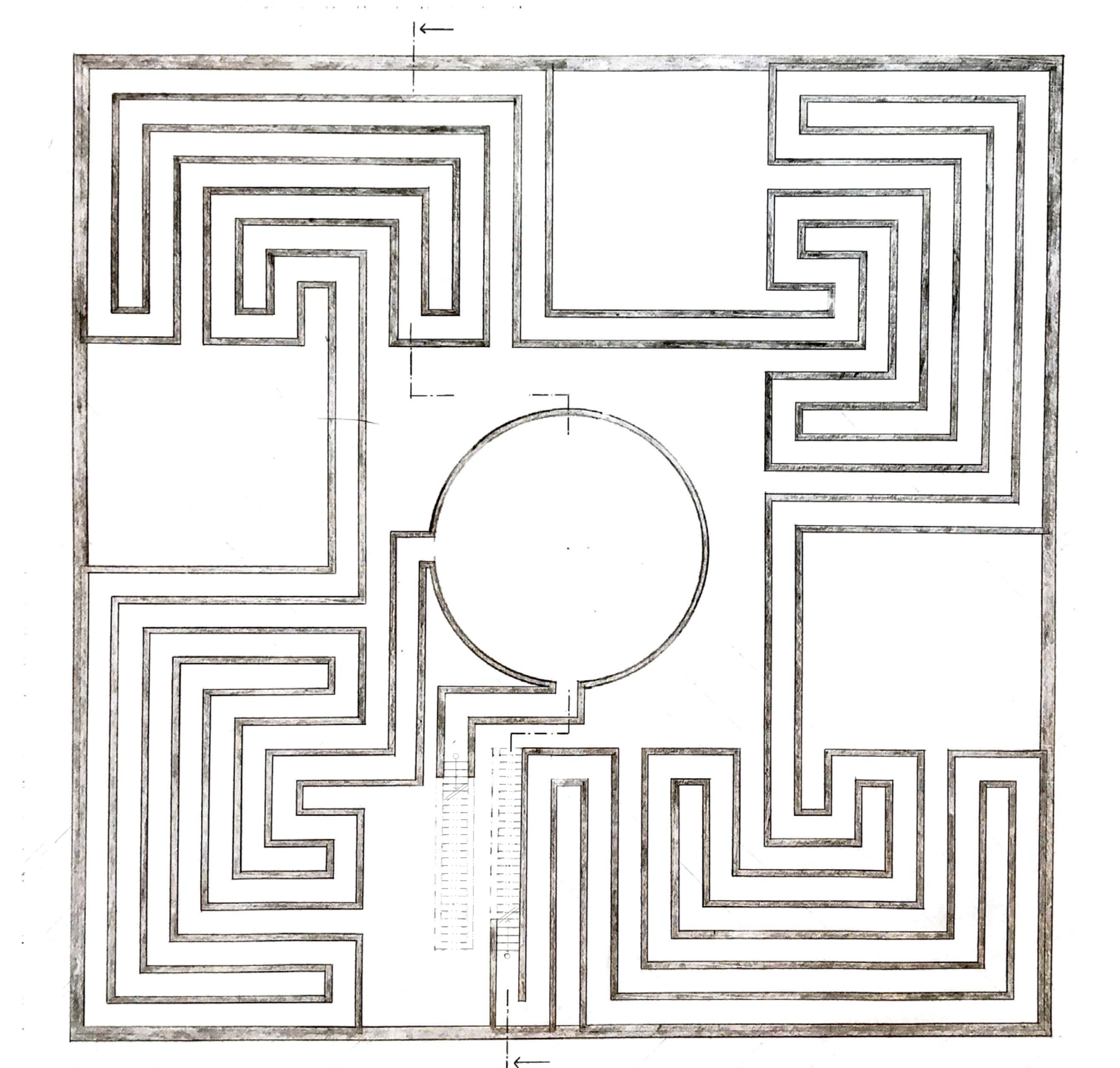
Púdorys Podzemí 1:100
