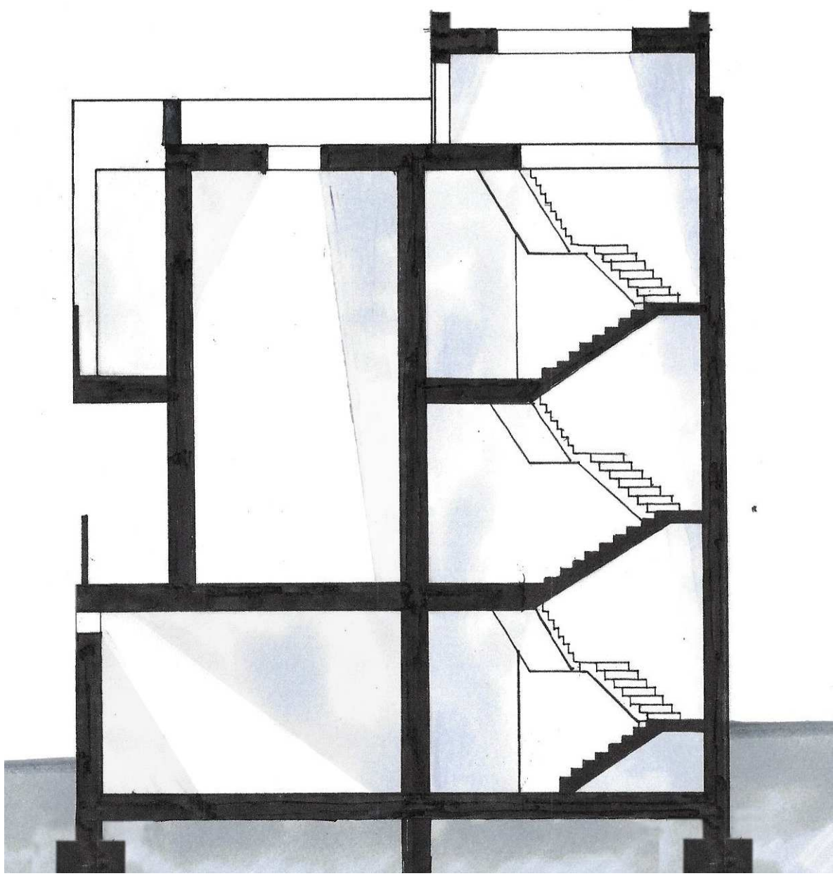
ŘEZ A-A' 1:100
