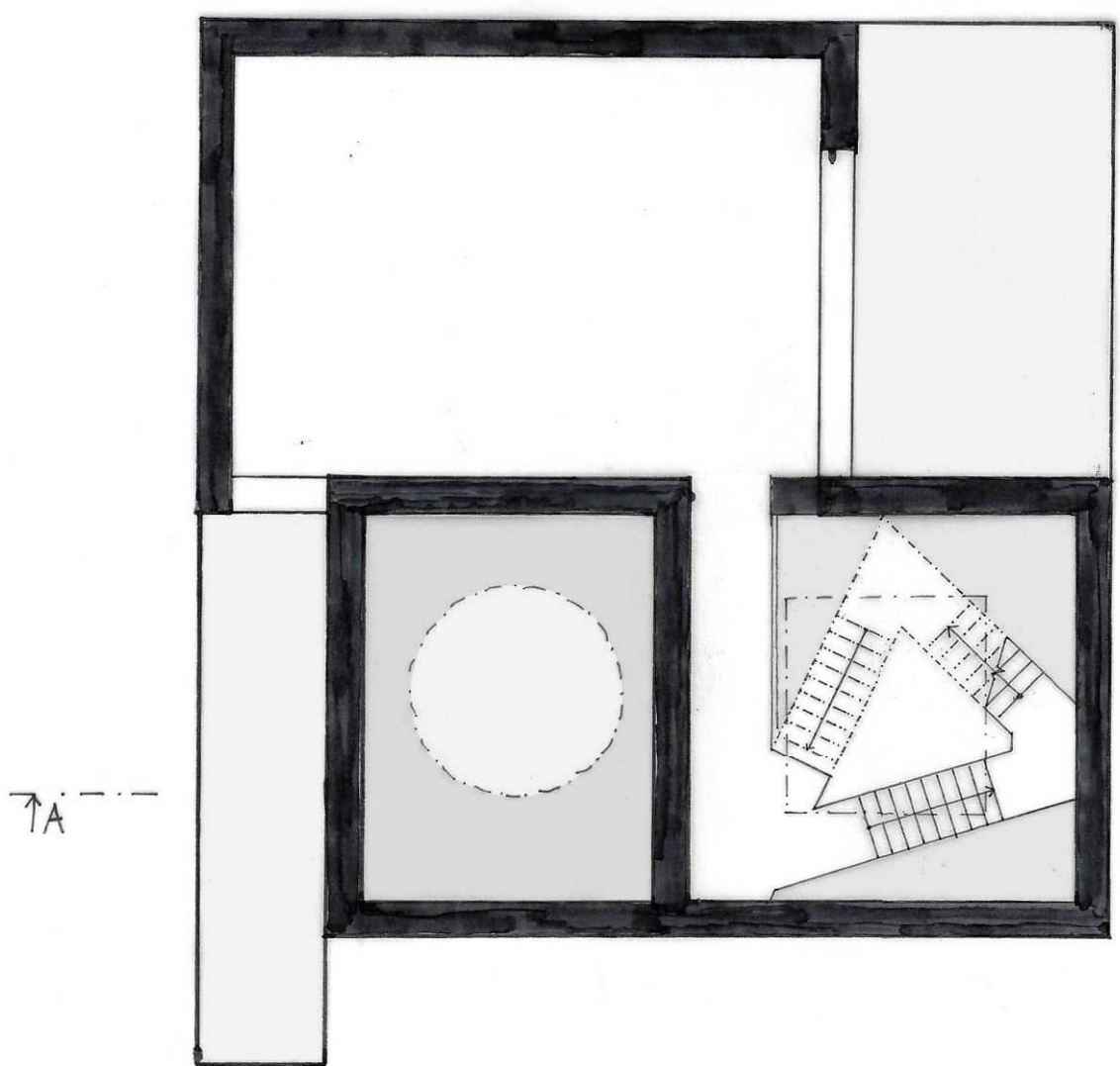
PŮDORYS 3NP 1:100
