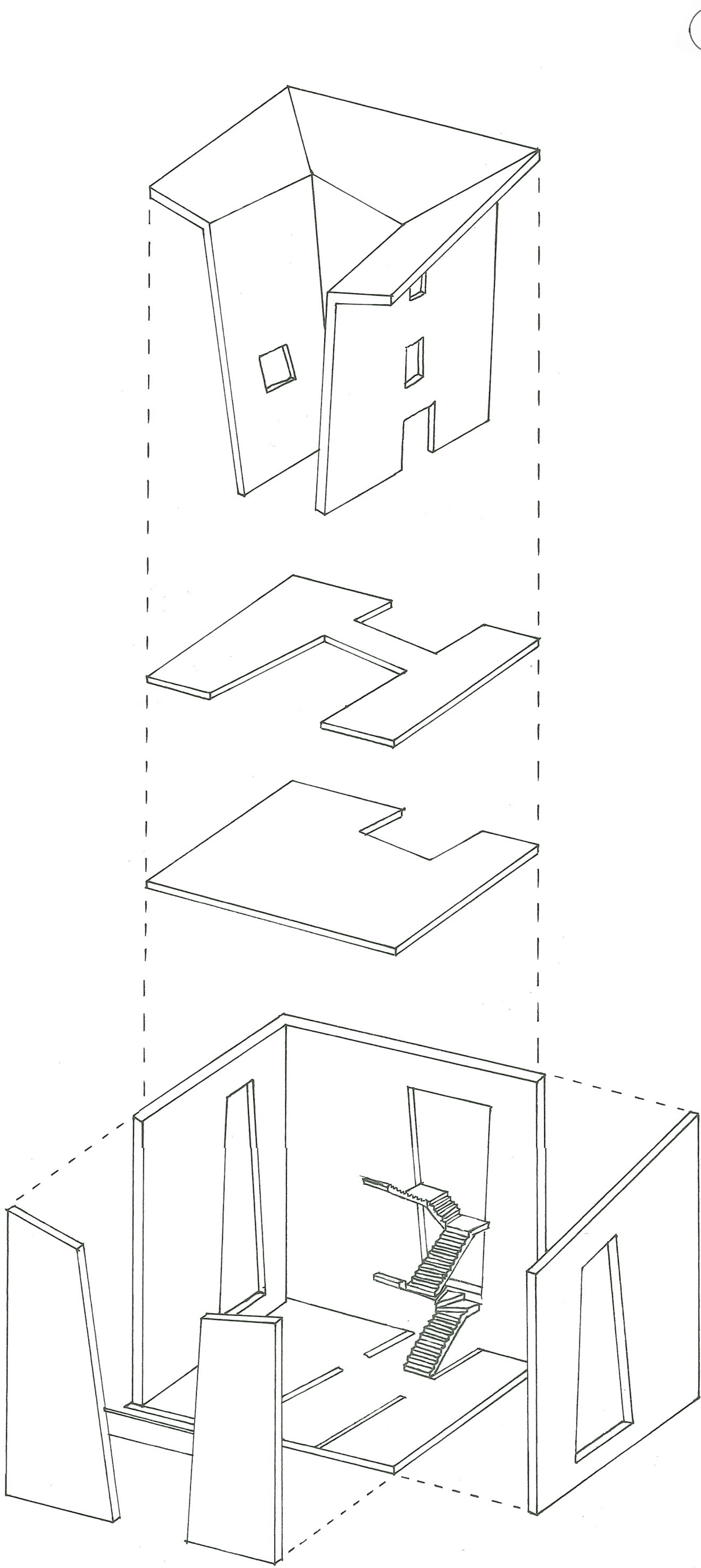
AXONOMETRIE
