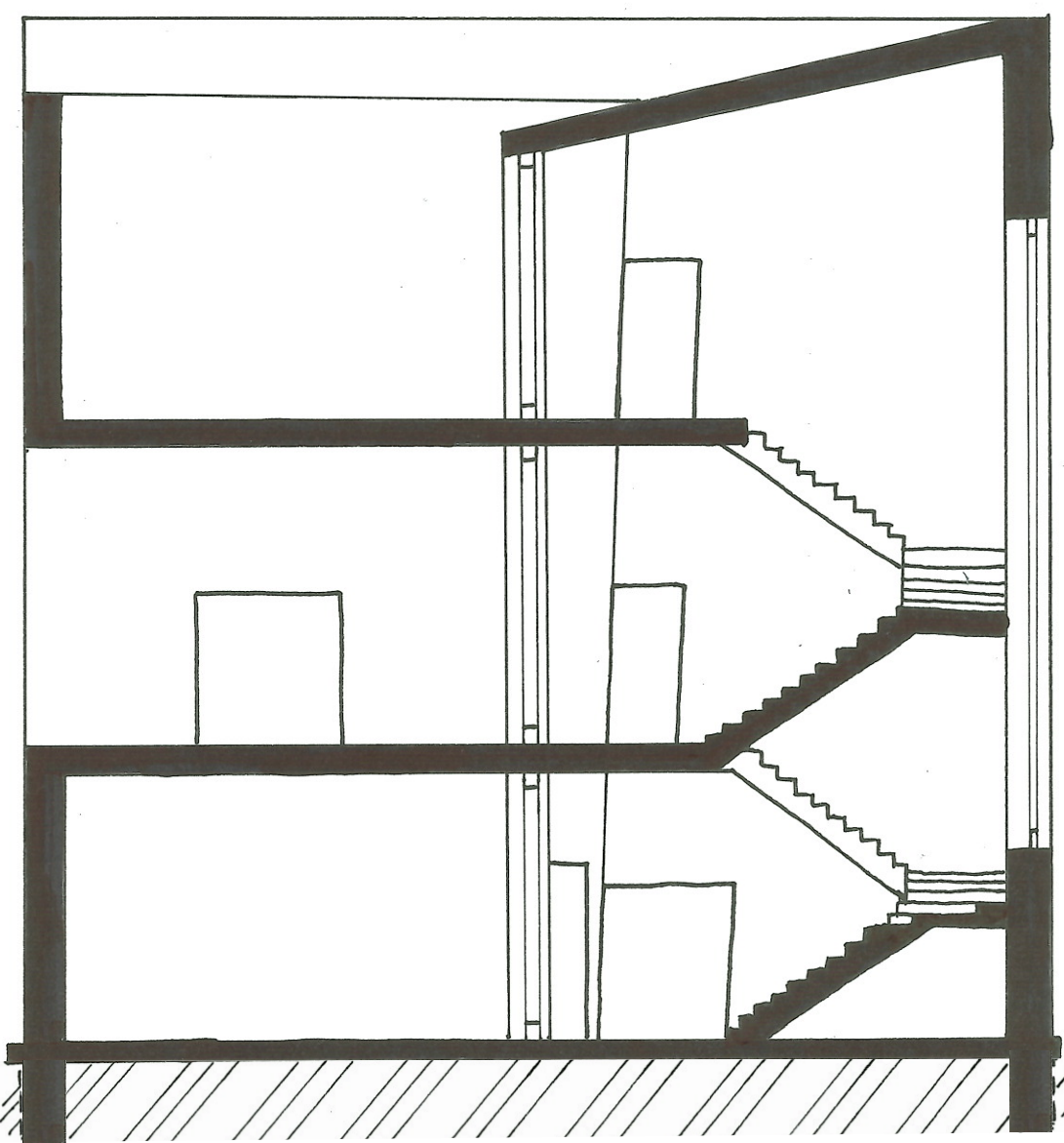
ŘEZ B-B 1:100
