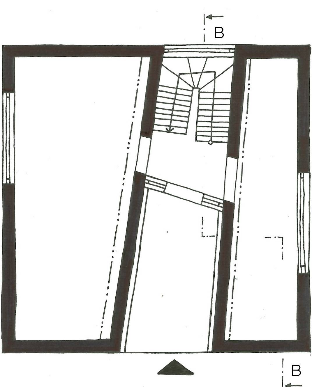
PŮDORYS 2NP 1:100
