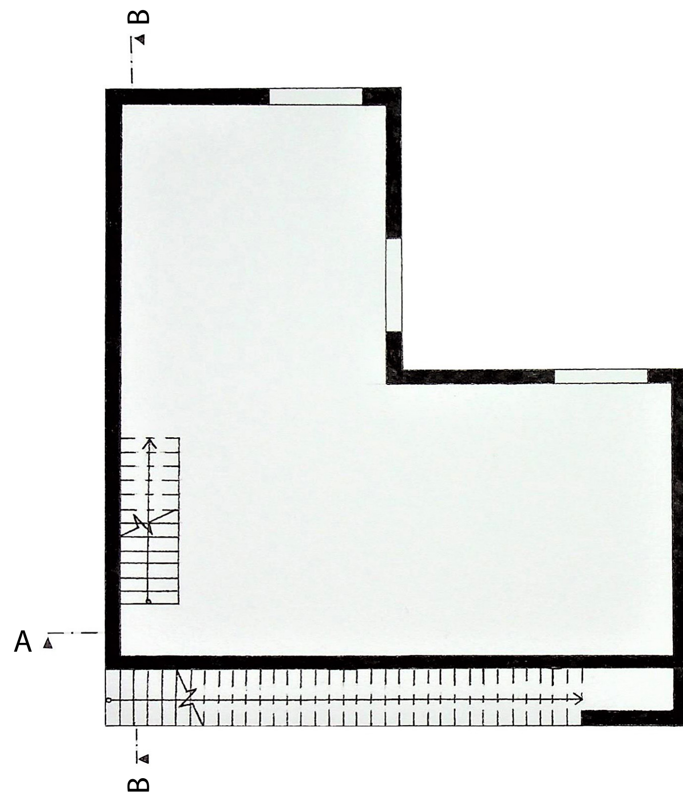
PŮDORYS 1NP
