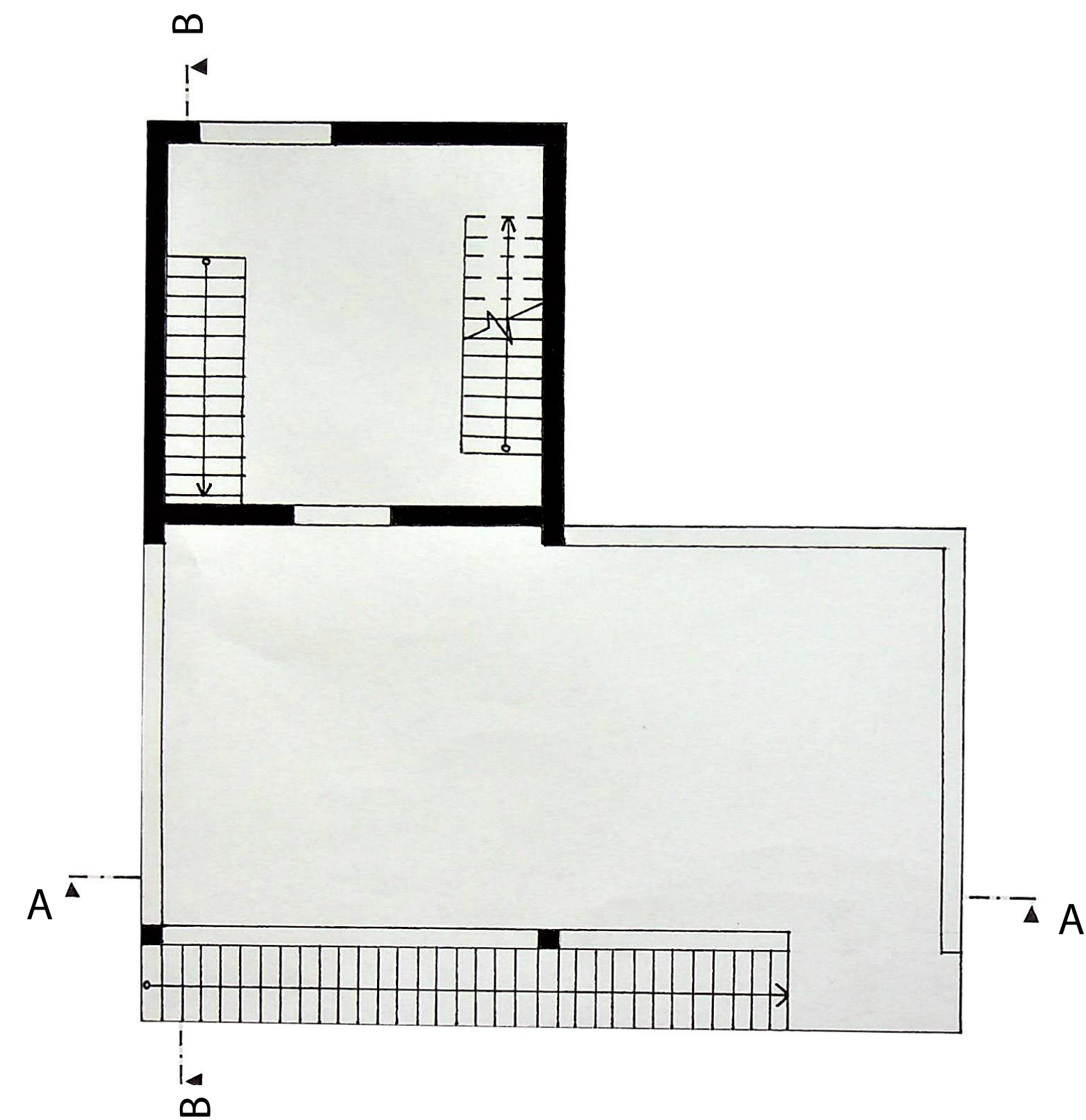
PŮDORYS 3NP
