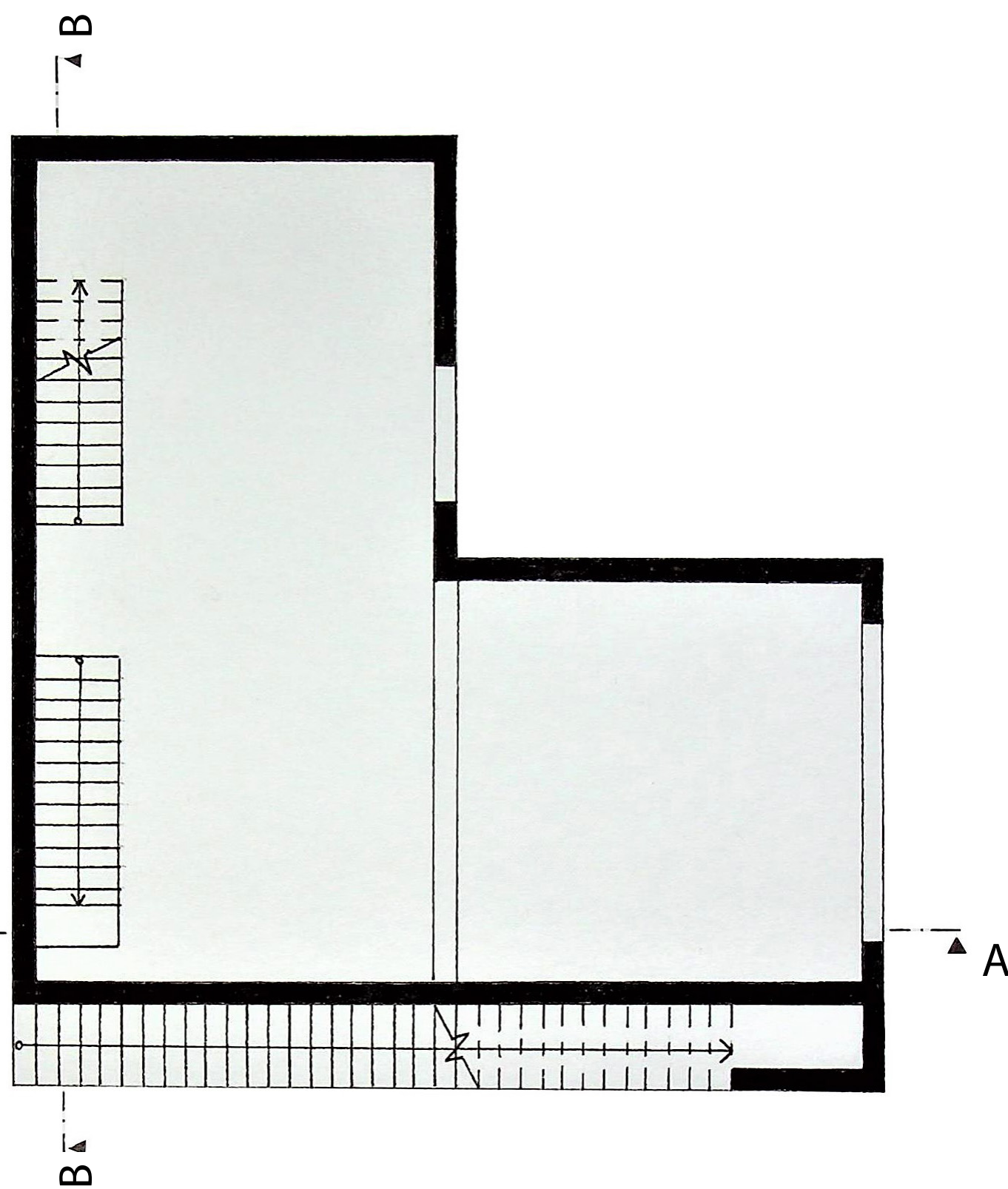
PŮDORYS 2NP
