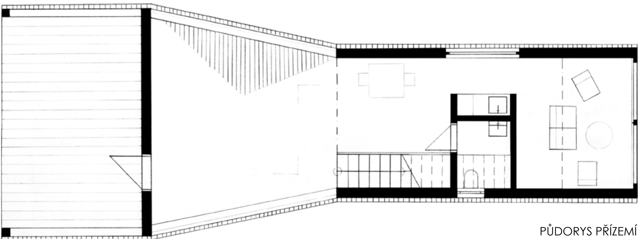
PŮDORYS PŘÍZEMÍ
