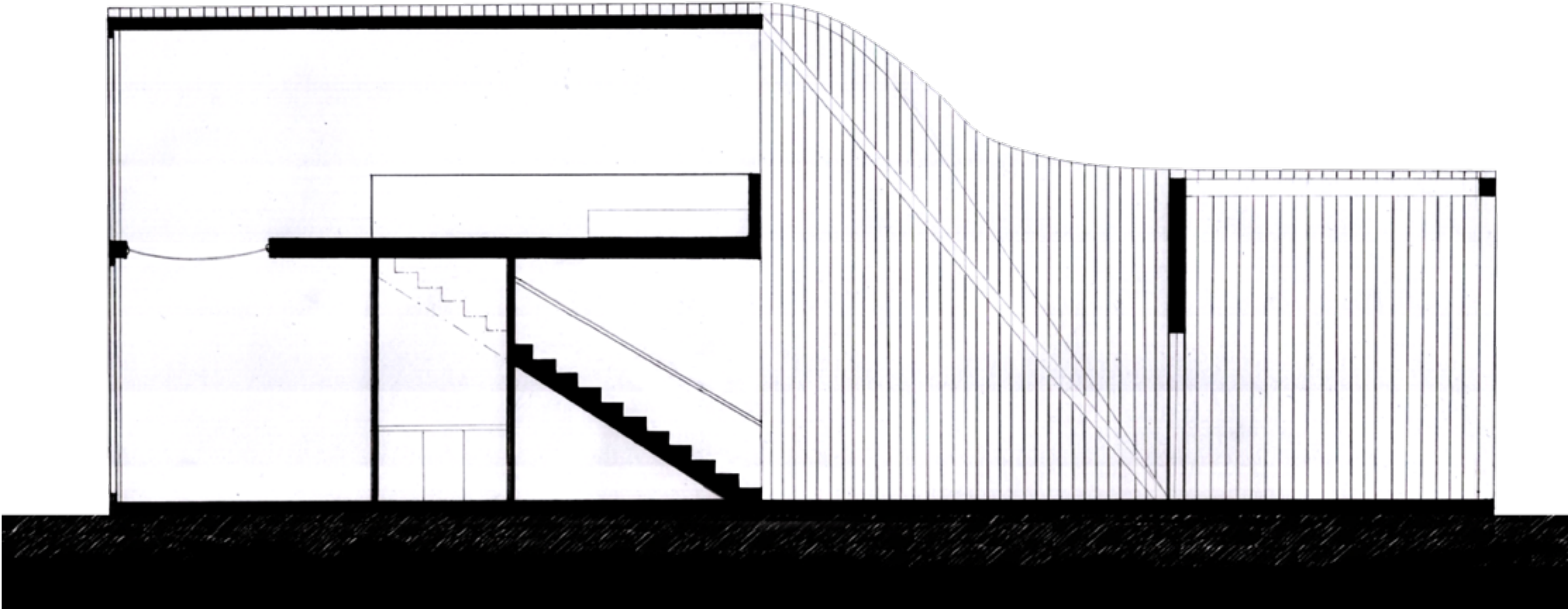
ŘEZ PODELNÝ
