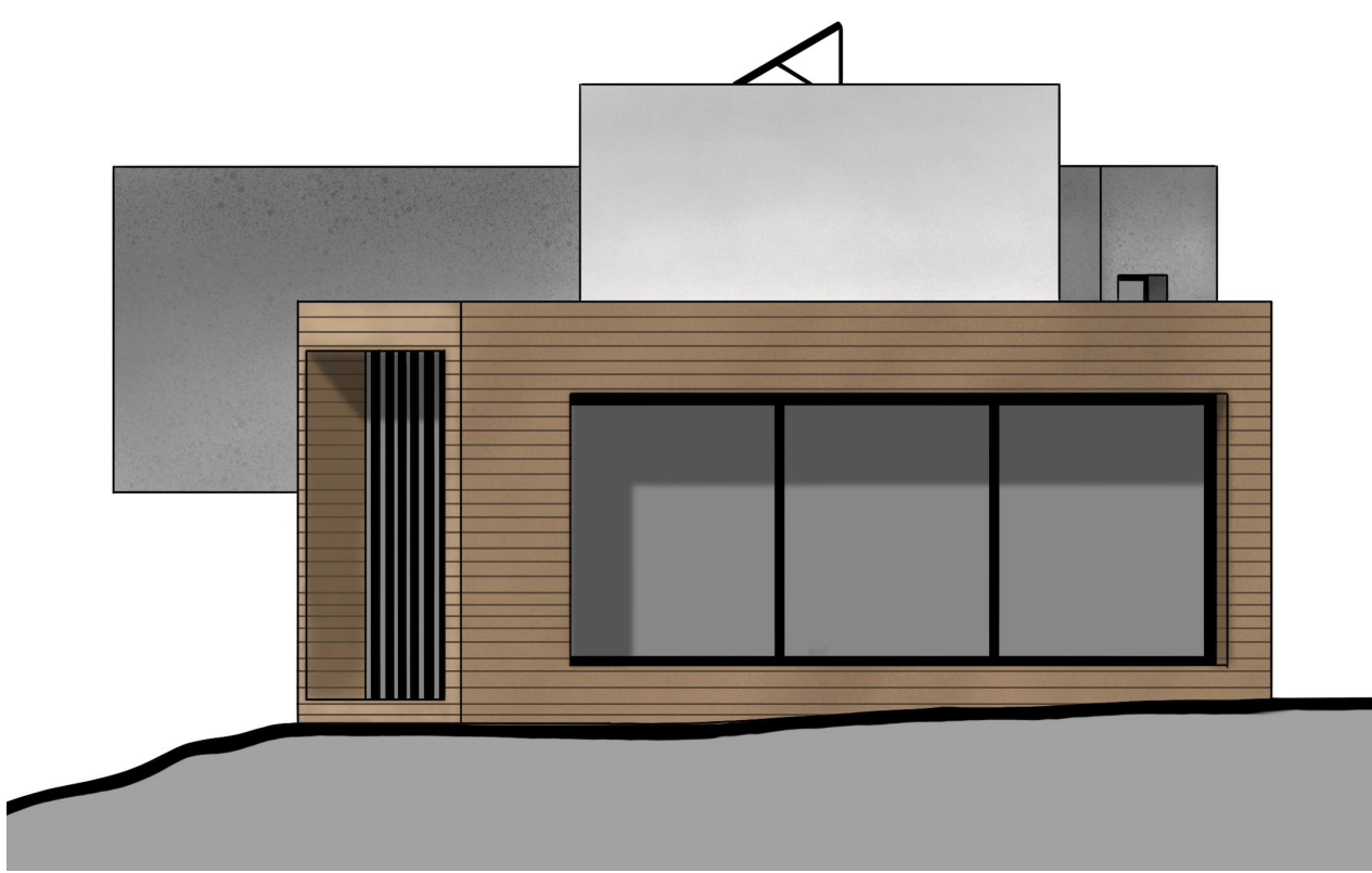
POHLED VÝCHODNÍ 1:100
