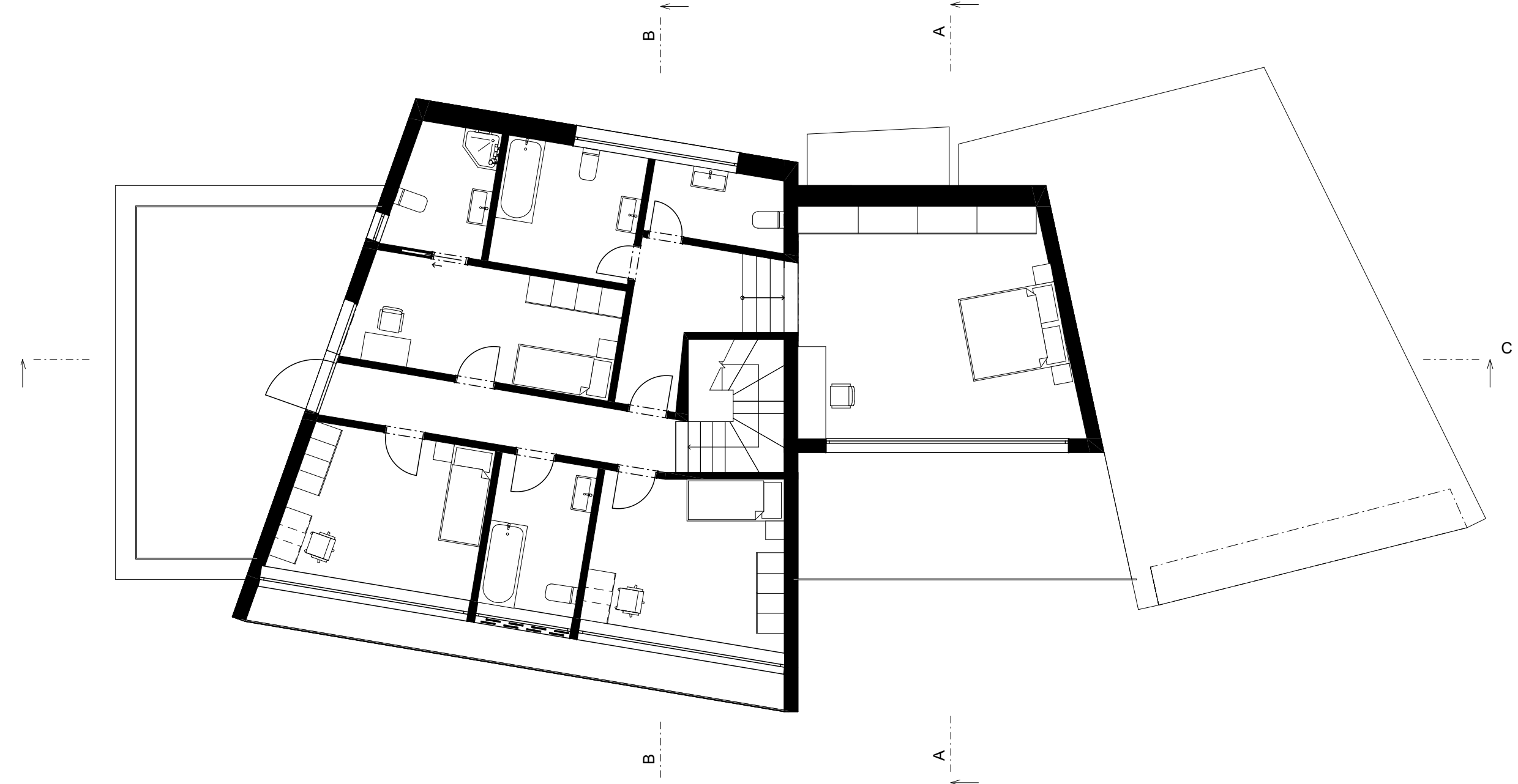
PŮDORYS 2NP 1:100
