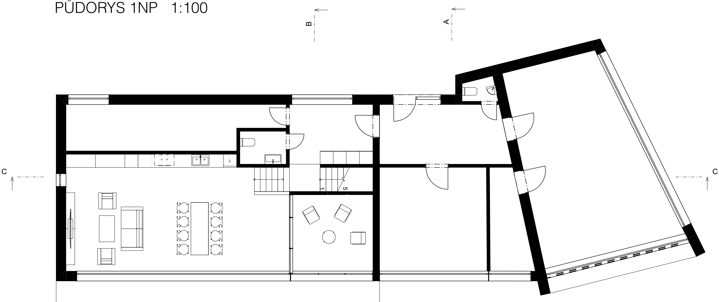
PŮDORYS 1NP 1:100
