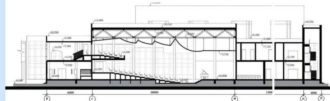
ŘEZ 2-2 (KLUB) M 1:500
