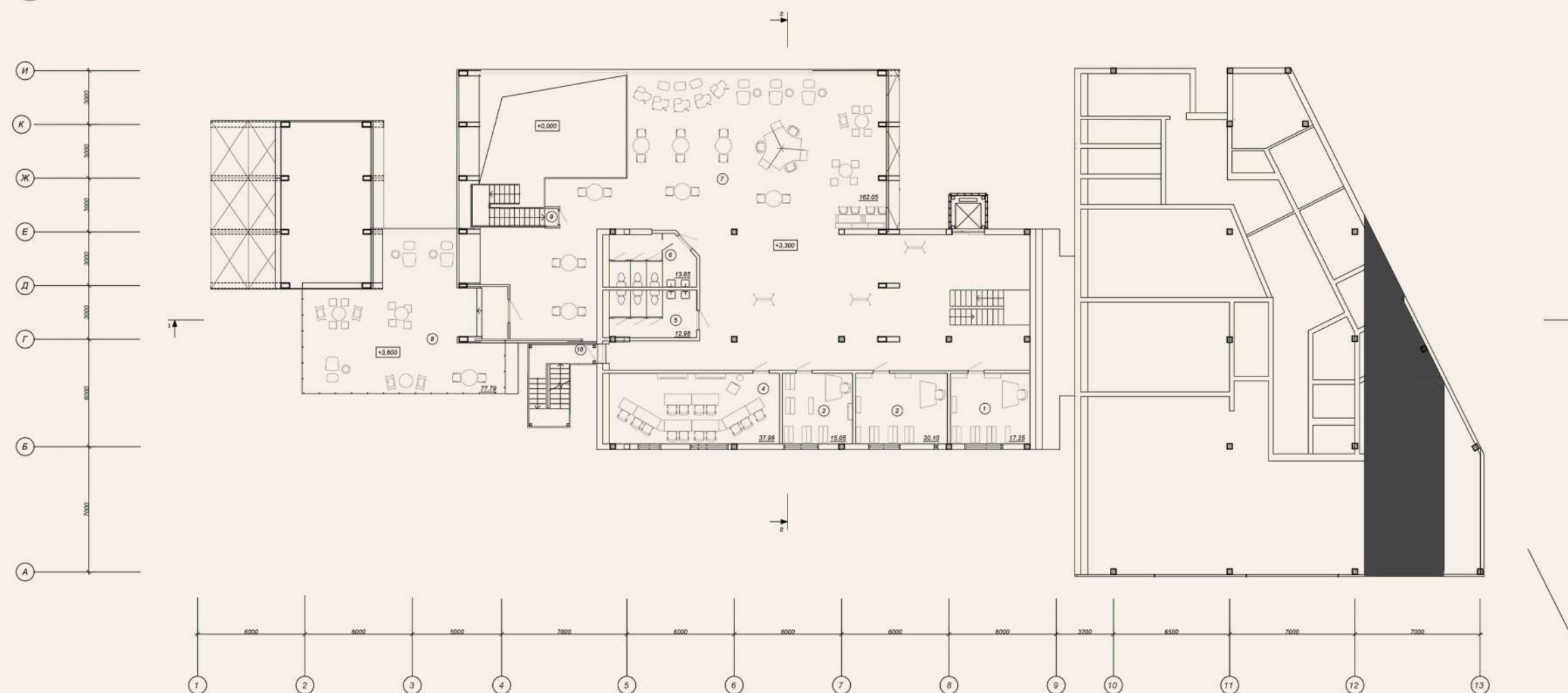
PŮDORYS 1.NP M 1:250
