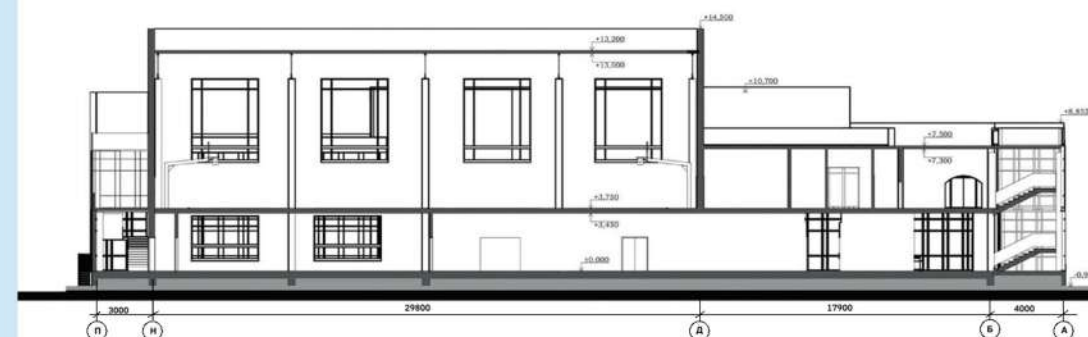
ŘEZ 3-3 (VYVOJOVÝ CENTRUM) M 1:500
