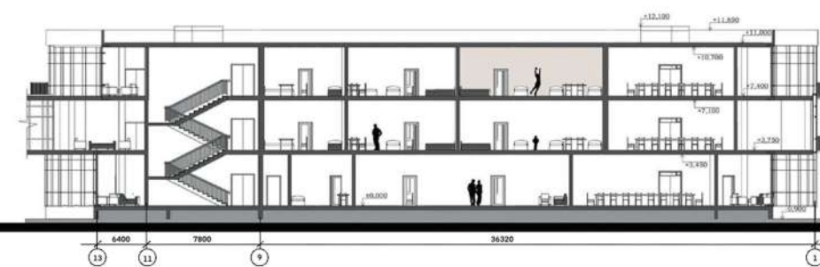
ŘEZ 4-4 (OBYTNÉ KŘÍDLO) M 1:500
