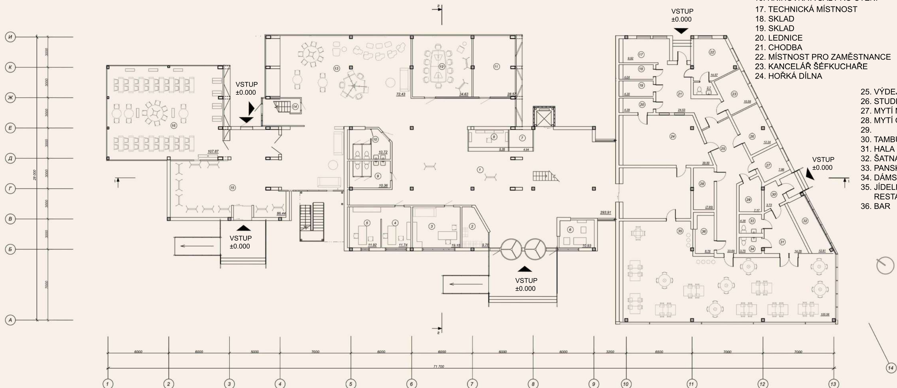
PŮDORYS 1.NP M 1:250
