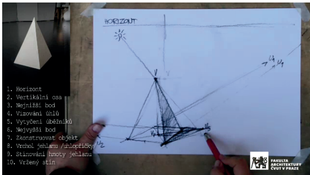
PERSPEKTIVA A STÍNOVÁNÍ JEHLANU
