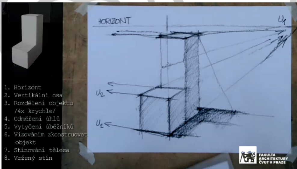
PERSPEKTIVA A STÍNOVÁNÍ PRAVOÚHLÉHO OBJEKTU
